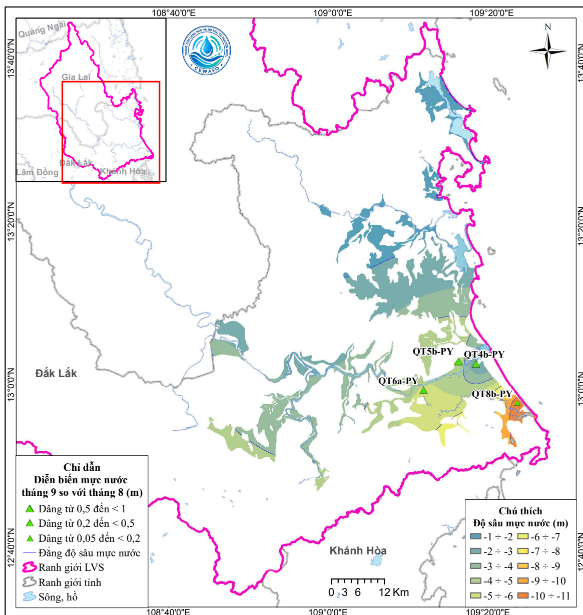
Hình 8. Sơ đồ diễn biến mực nước tháng 9 tăng q
