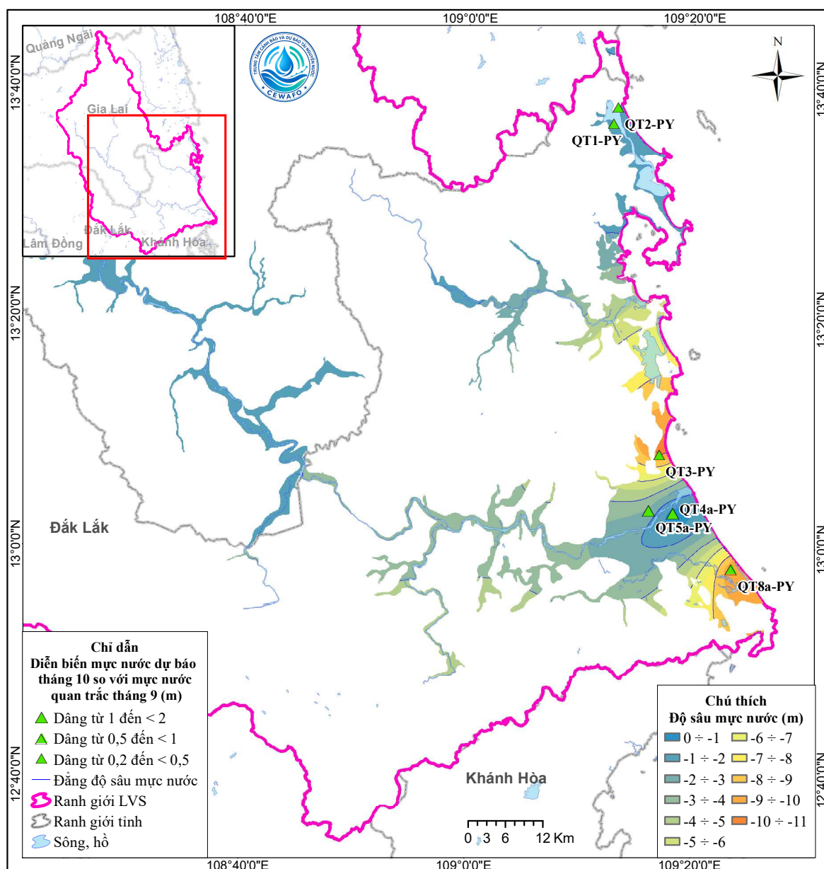
Hình 17. Sơ đồ dự báo diễn biến mực nước tháng 10 tầng qh
