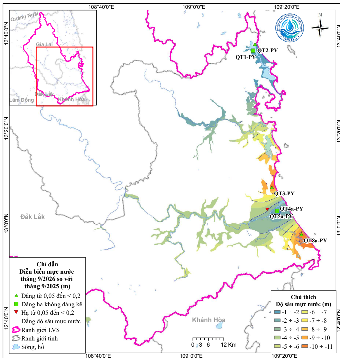
Hình 7. Sơ đồ diễn biến mực nước tháng 9 so với cùng kỳ năm trước
