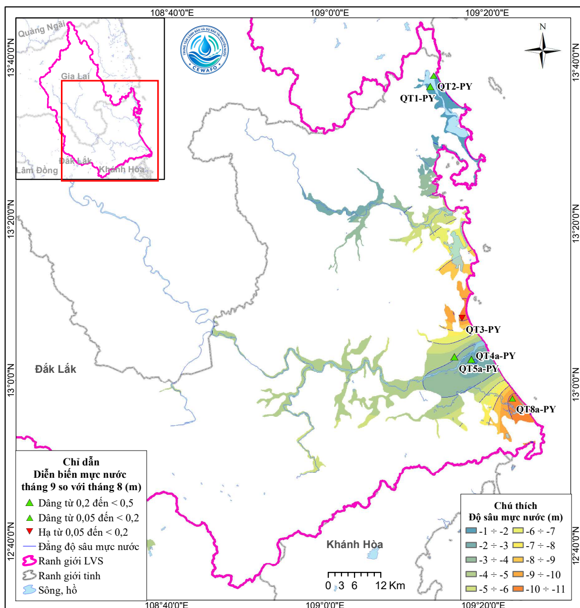
Hình 6. Sơ đồ diễn biến mực nước tháng 9 tầng qh
