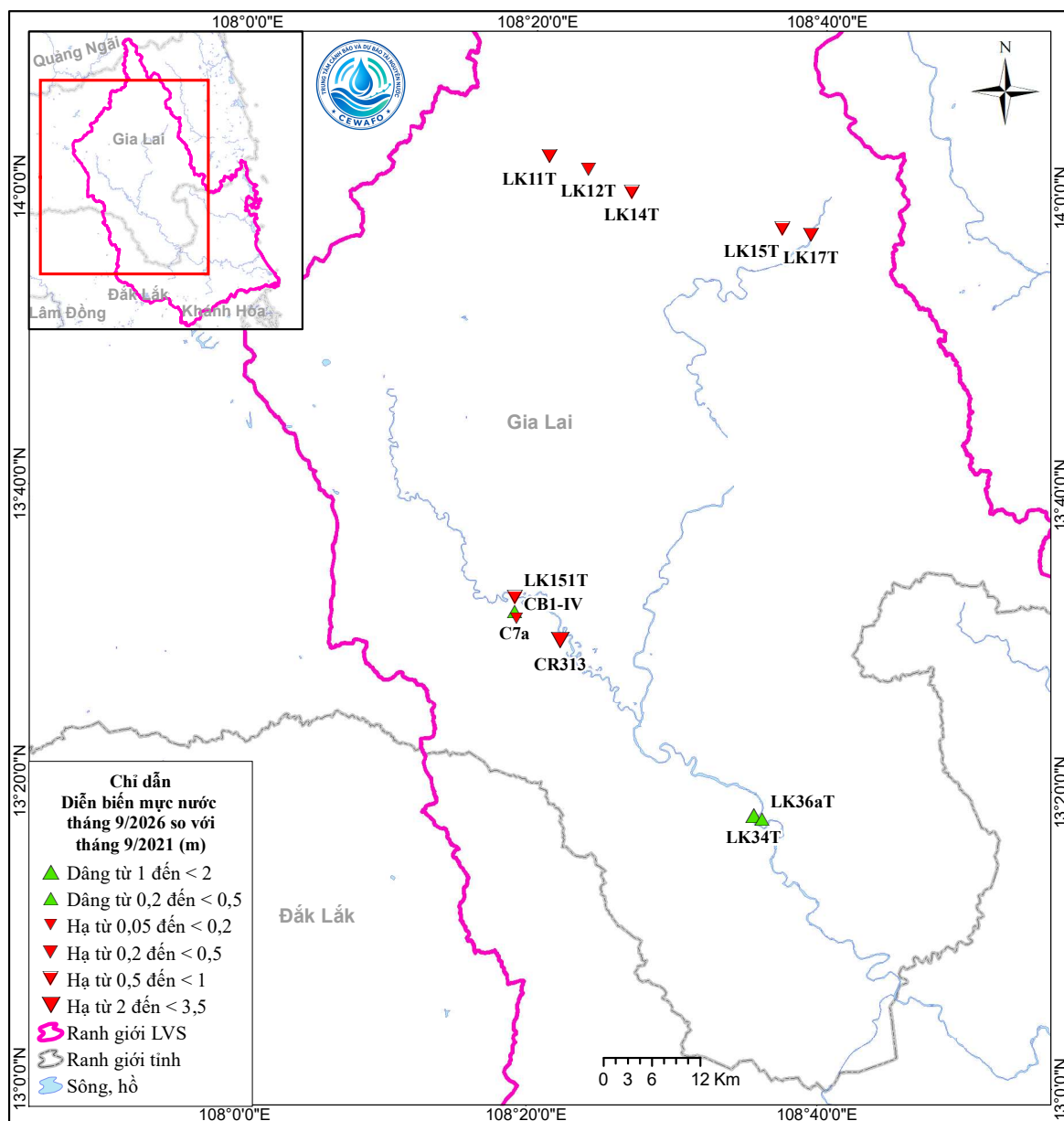
Hình 5. Sơ đồ diễn biến mực nước tháng 9 so với cùng kỳ 5 năm trước
