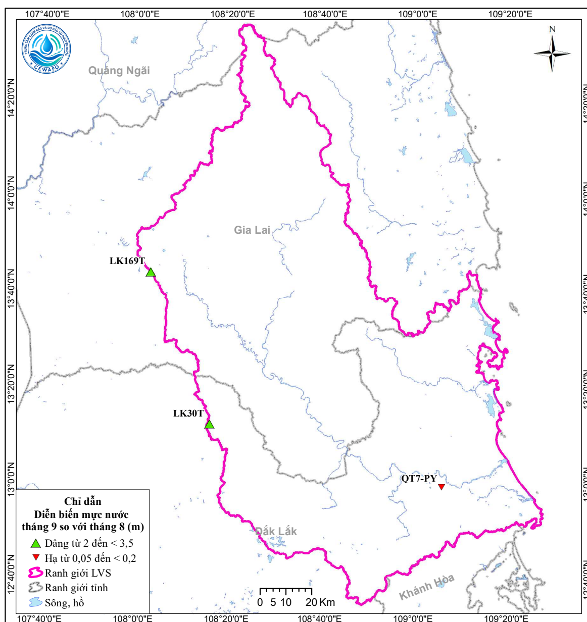
Hình 10. Sơ đồ diễn biến mực nước tháng 9 tầng \beta(n_2-qp)
