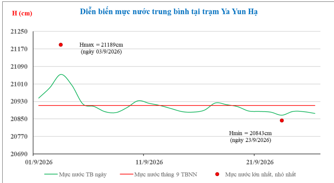
Hình 2. Diễn biến mức nước trung bình ngày tháng 9 năm 2026 tại trạm Ya Yun Hạ
