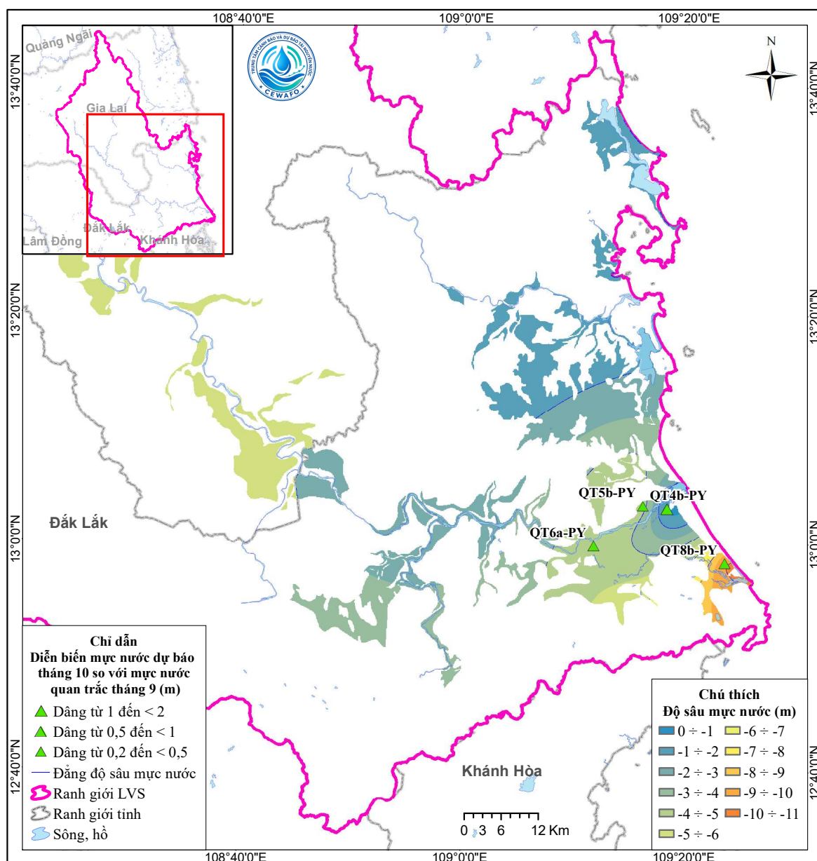
Hình 18. Sơ đồ dự báo diễn biến mực nước tháng 10 tầng qp
