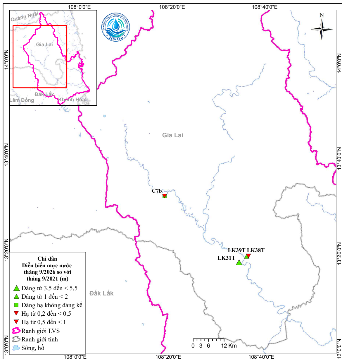
Hình 15. Sơ đồ diễn biến mực nước tháng 9 so với cùng kỳ 5 năm trước
