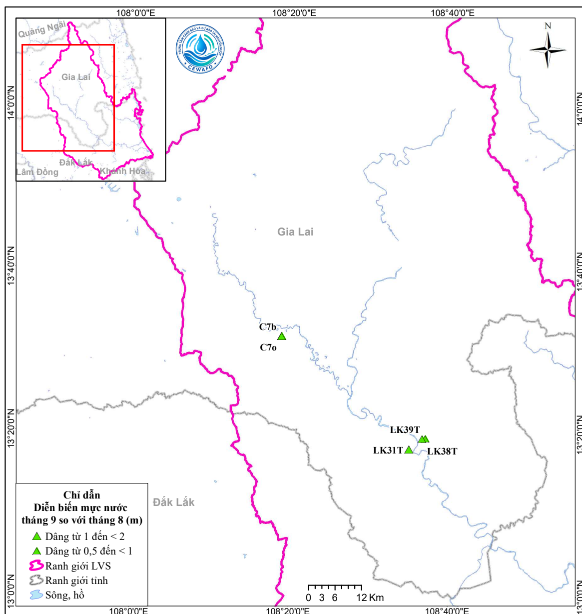
Hình 13. Sơ đồ diễn biến mực nước tháng 9 tăng n
