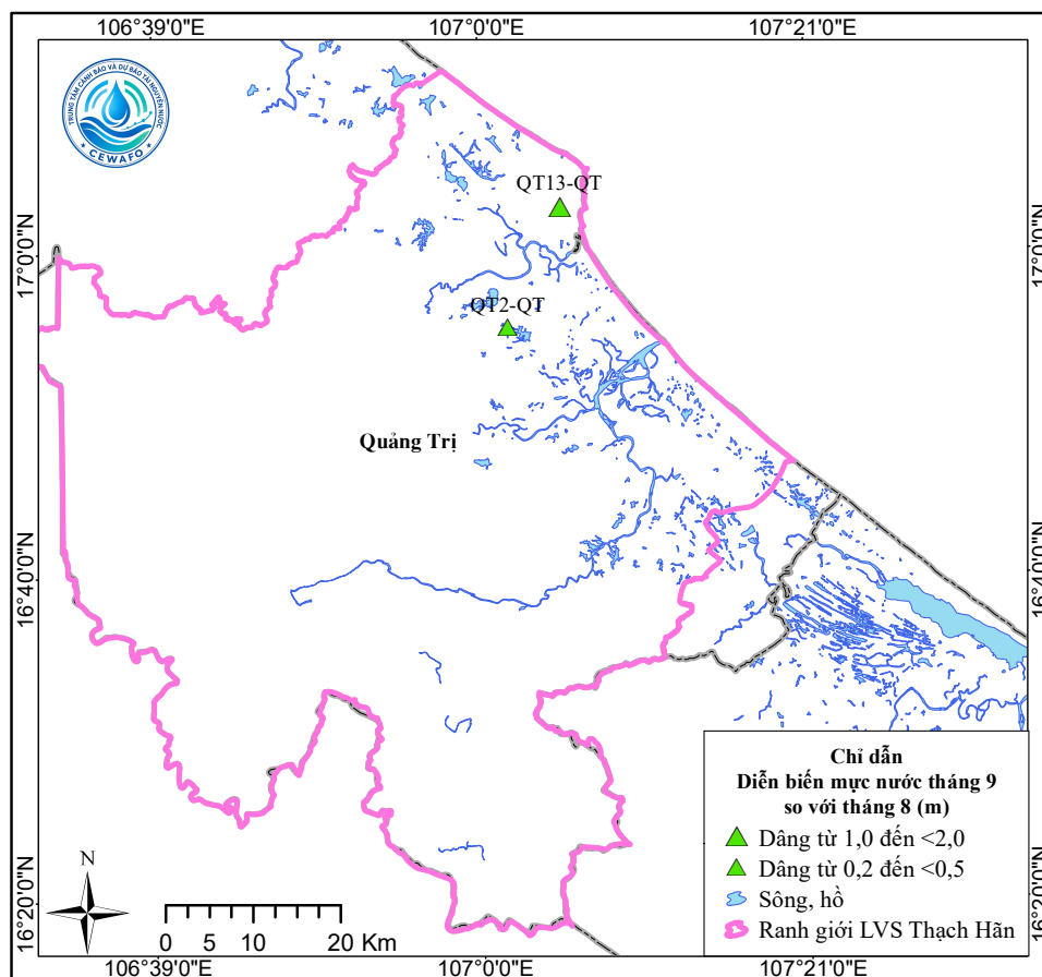
Hình 10. Sơ đồ diễn biến mực nước tháng 9 tầng \beta(n-q)
