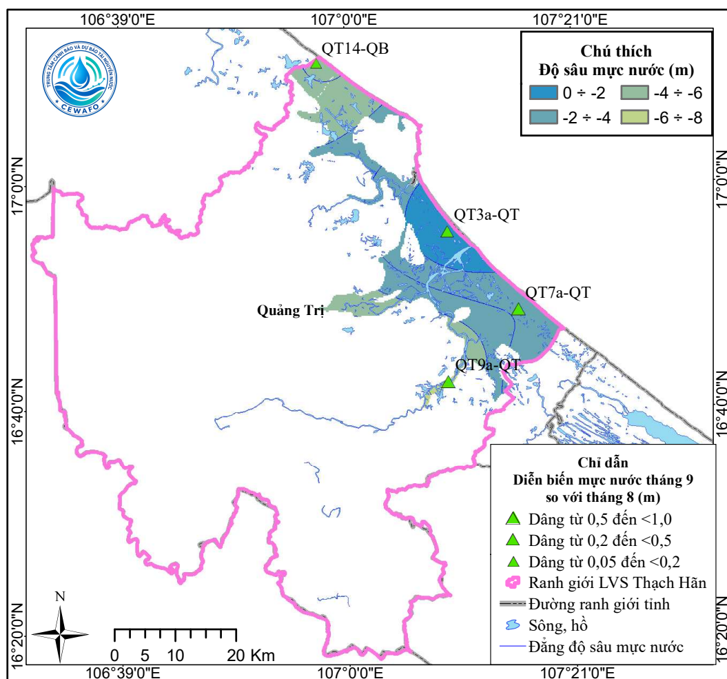
Hình 1. Sơ đồ diễn biến mực nước tháng 9 tăng qh
