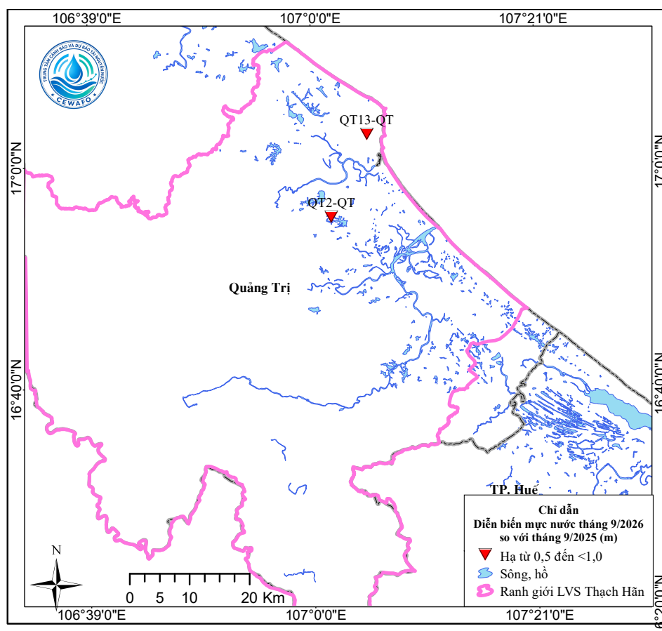
Hình 11. Sơ đồ diễn biến mực nước tháng 9 so với cùng kỳ năm trước
