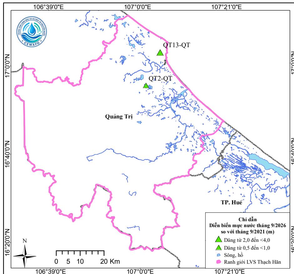
Hình 12. Sơ đồ diễn biến mực nước tháng 9 so với cùng kỳ 5 năm trước 1.2.2.5. Tầng chứa nước khe nứt trong đá trầm tích lục nguyên Devon dưới
