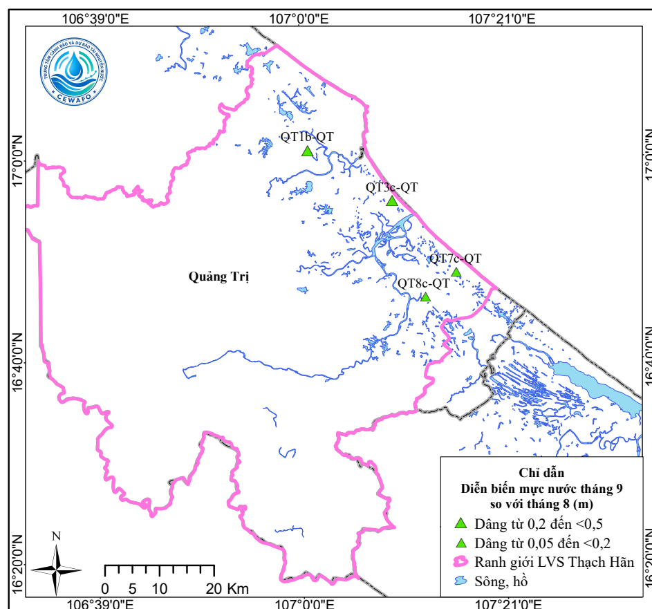
Hình 7. Sơ đồ diễn biến mực nước tháng 9 tầng n
