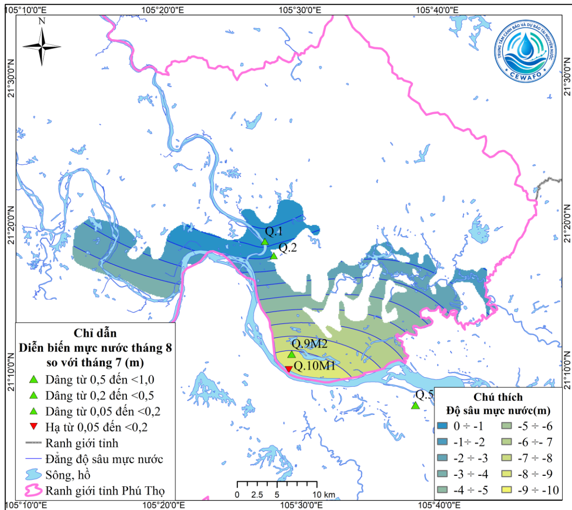
Hình 1. Sơ đồ diễn biến mực nước lớp q_2
