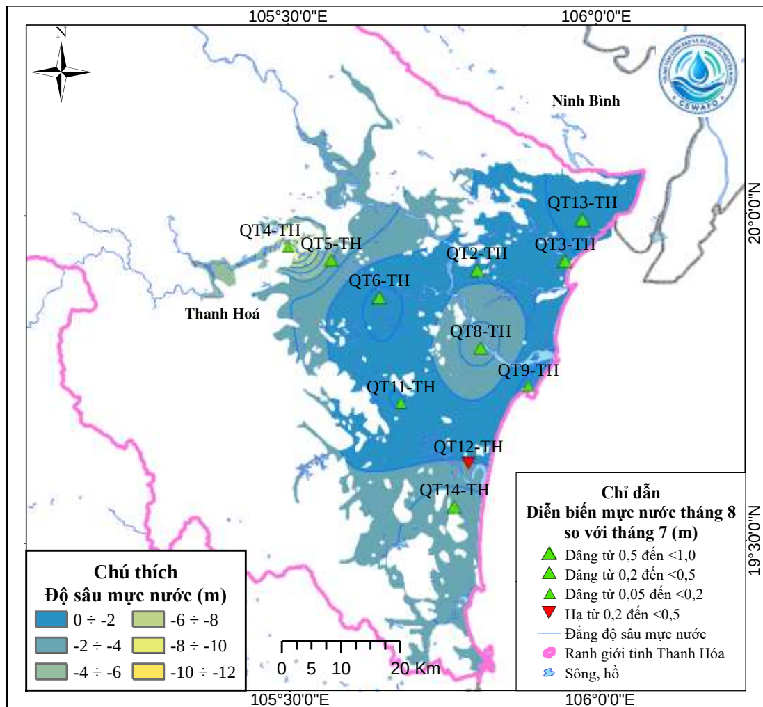
Hình 1. Sơ đồ diễn biến mực nước tháng 8 tăng qh
