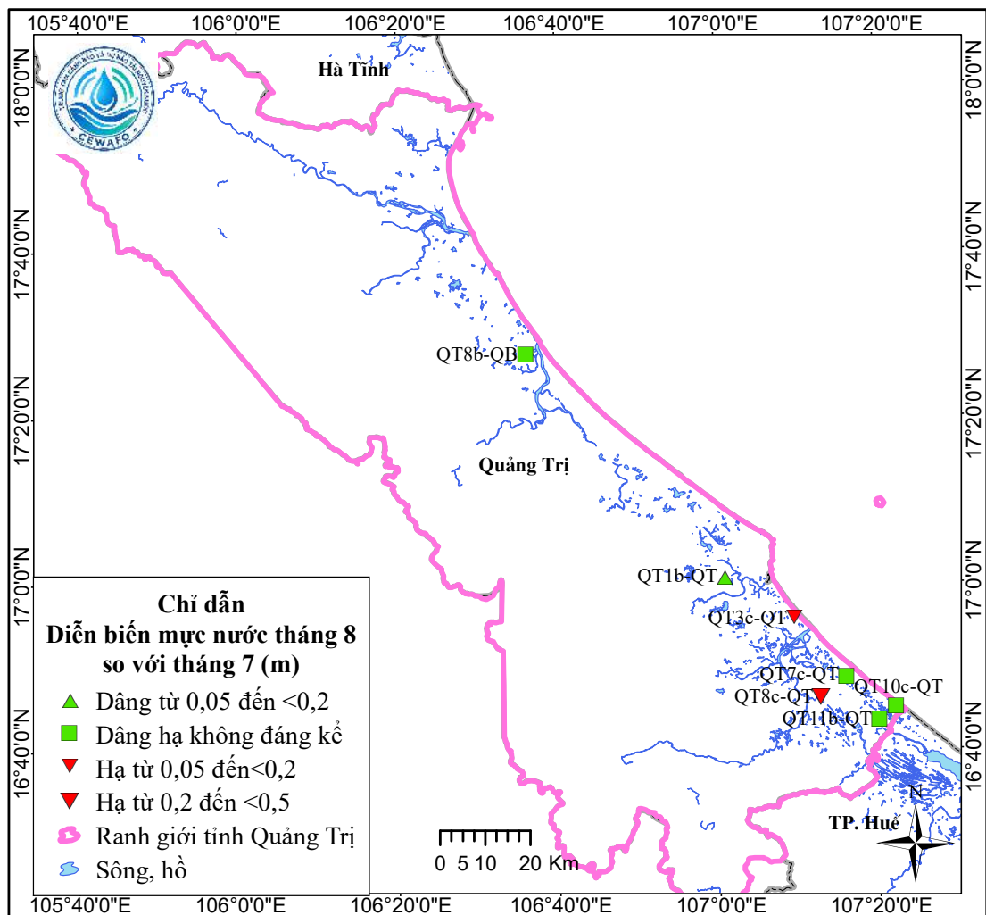
Hình 3. Sơ đồ diễn biến mực nước tháng 8 tầng n
