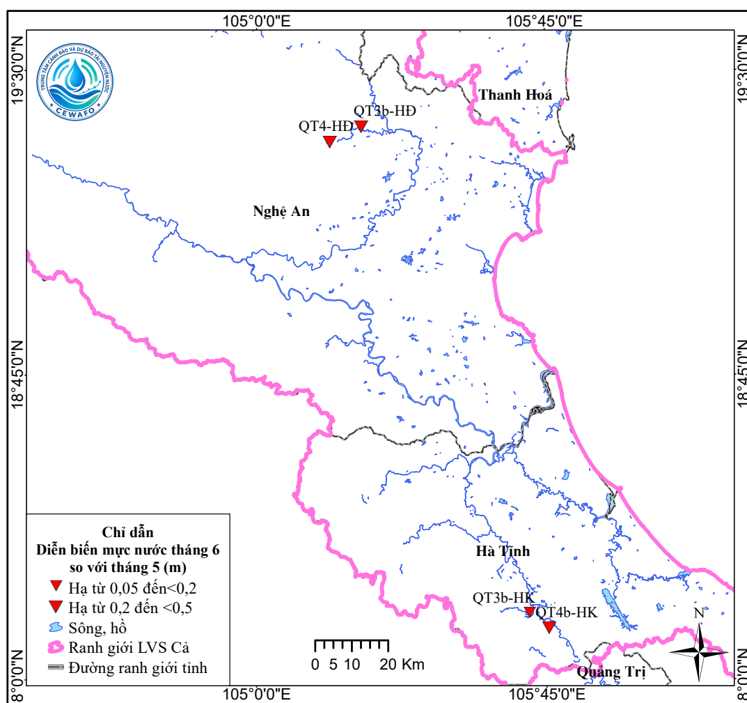
Hình 10. Sơ đồ diễn biến mực nước tháng 6 tầng c-p
