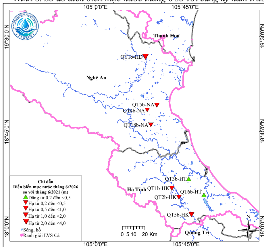
Hình 9. Sơ đồ diễn biến mực nước tháng 6 so với cùng kỳ 5 năm trước
