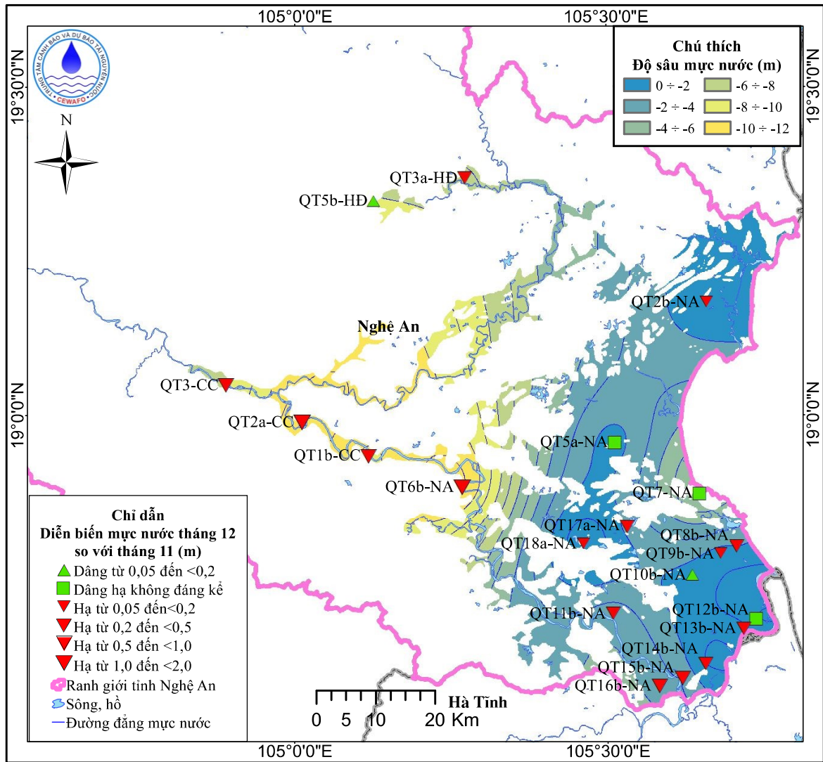
Hình 2. Sơ đồ diễn biến mực nước tháng 12 tầng q p
