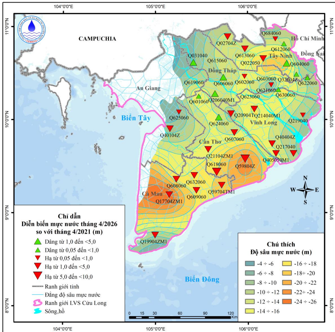
Hình 20. Sơ đồ diễn biến mực nước tháng 4 so với cùng kỳ 5 năm trước g) Tầng chứa nước lỗ hổng trong các đá trầm tích Miocene ( n_1^3 )
