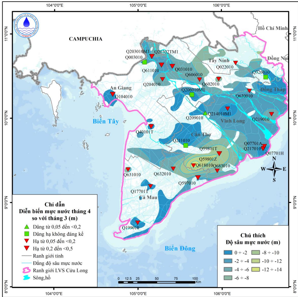
Hình 3. Sơ đồ diễn biến mực nước tháng 4 tầng qh
