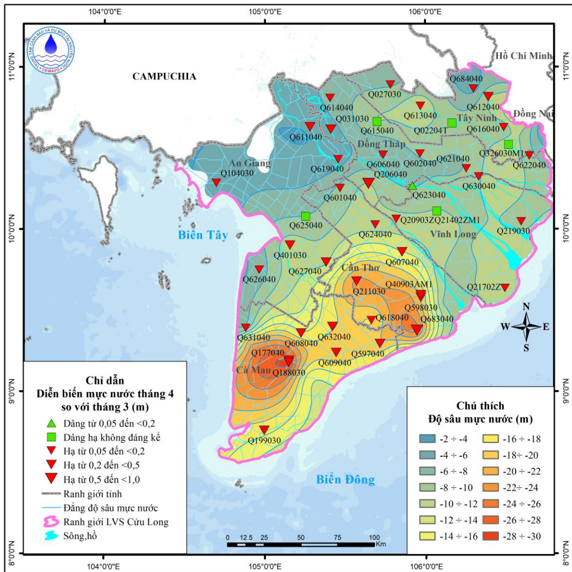
Hình 12. Sơ đồ diễn biến mực nước tháng 4 tầng q 1
