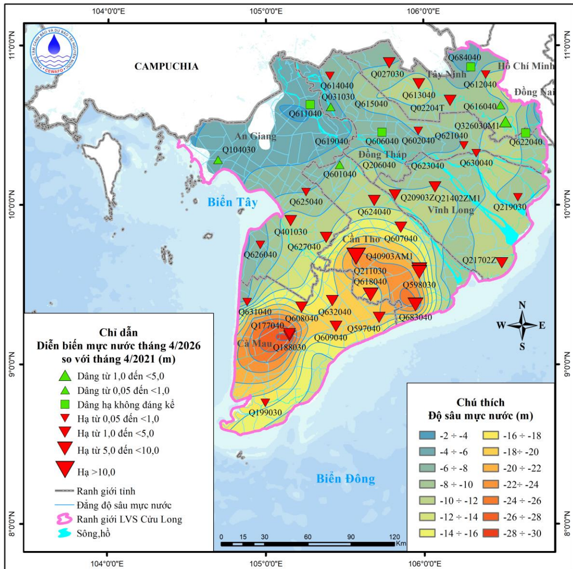
Hình 14. Sơ đồ diễn biến mực nước tháng 4 so với cùng kỳ 5 năm trước e) Tầng chứa nước lỗ hổng trong các đá trầm tích Pliocene giữa ( n_2^2 )
