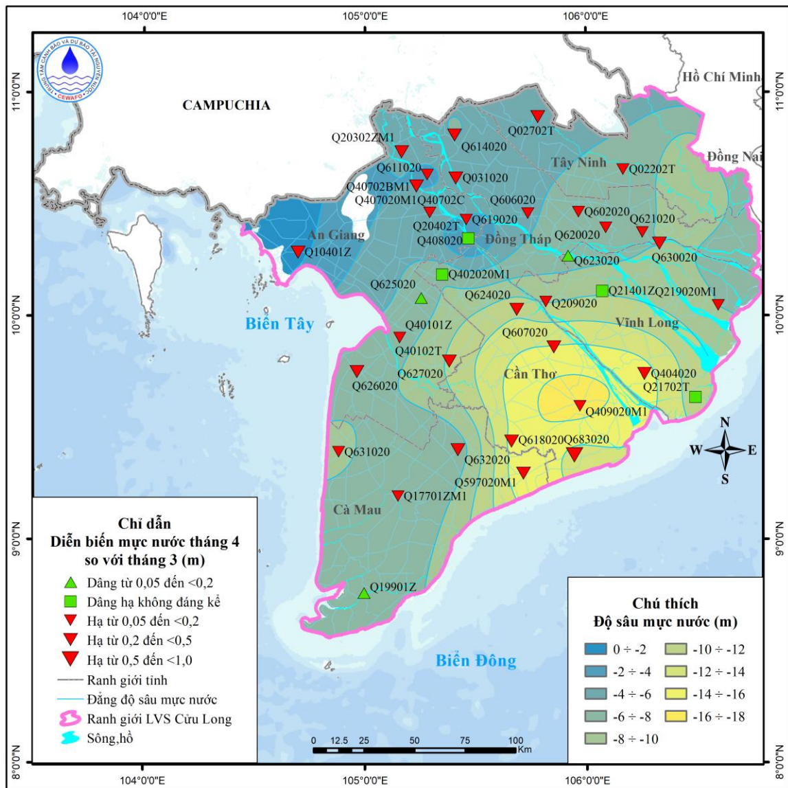
Hình 6. Sơ đồ diễn biến mực nước tháng 4 tầng q 3
