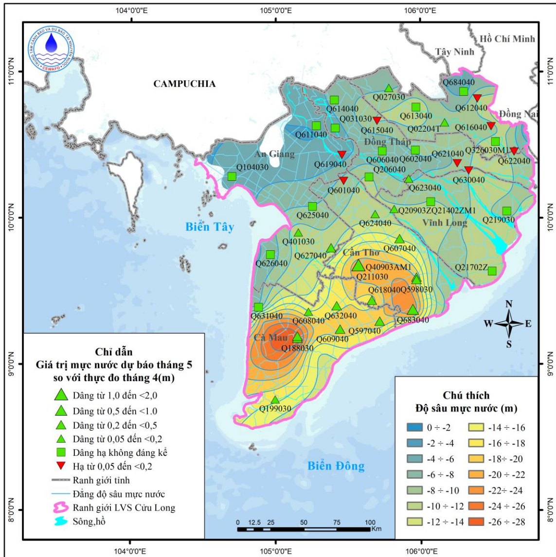
Hình 30. Sơ đồ dự báo diễn biến mực nước tầng qp_1 tháng 5 năm 2026
