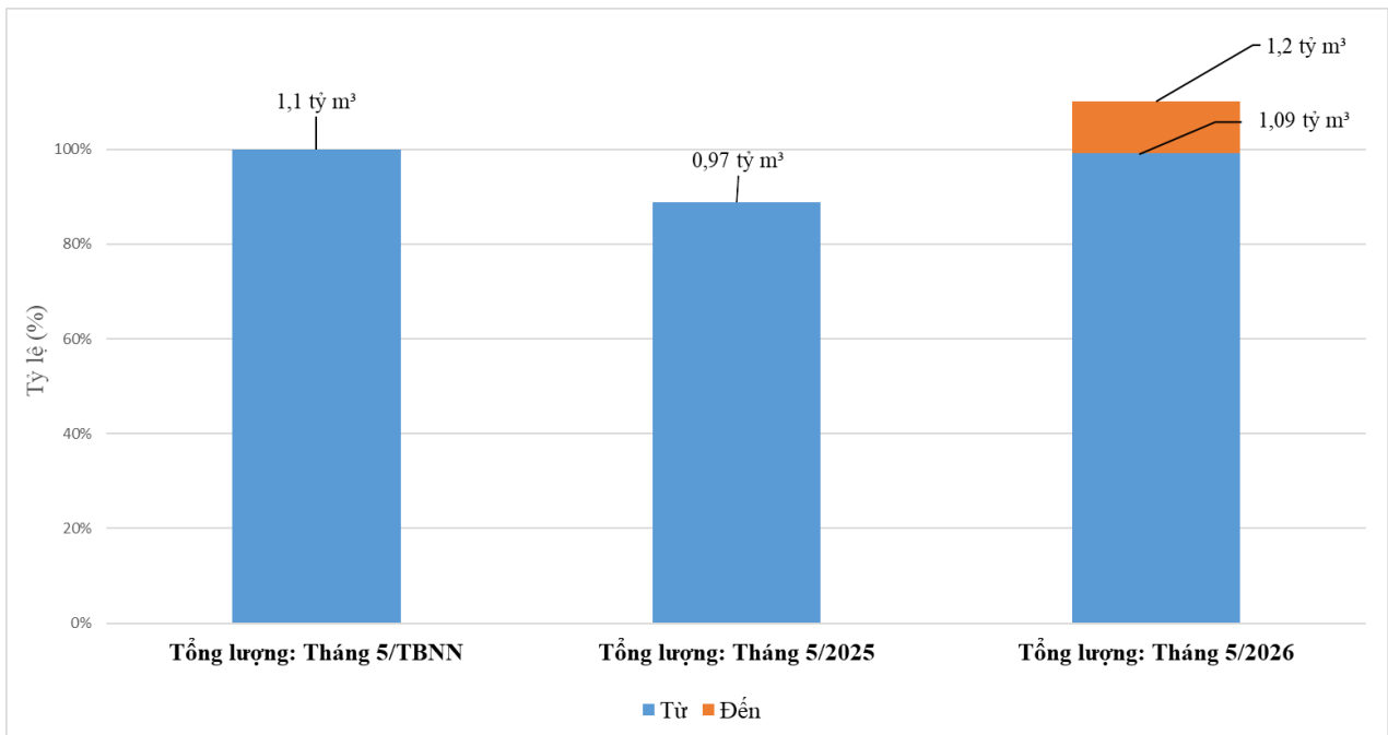
Hình 25. Biểu đồ tỷ lệ tổng lượng nước dự báo của lưu vực sông Cừ Long trong tháng 5 năm 2026 so với tháng cùng kỳ năm trước và tháng 5 TBNN
