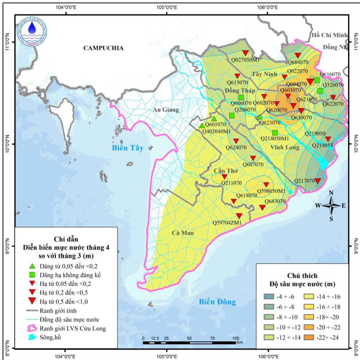
Hình 21. Sơ đồ diễn biến mực nước tháng 4 tầng n 3
