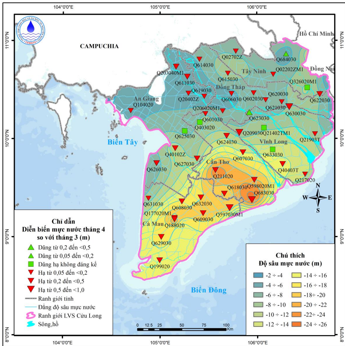
Hình 9. Sơ đồ diễn biến mực nước tháng 4 tầng qp2-3
