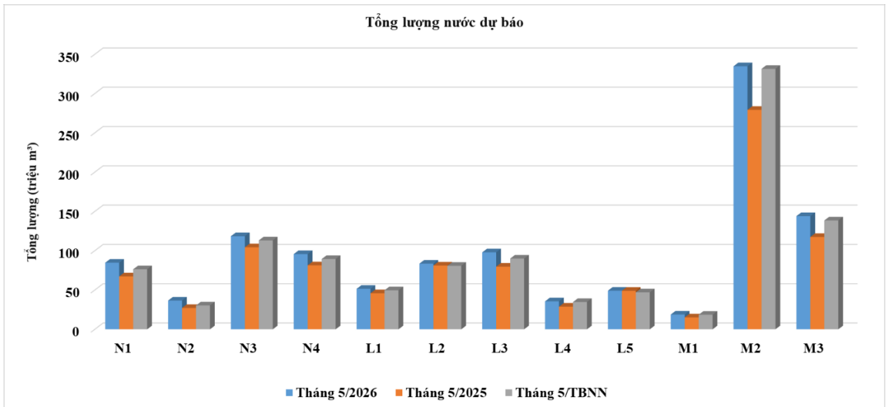
Hình 24. Biểu đồ tổng lượng nước dự báo của các tiểu vùng trong tháng 5 năm 2026 so với tháng cùng kỳ năm trước và tháng 5 TBNN
