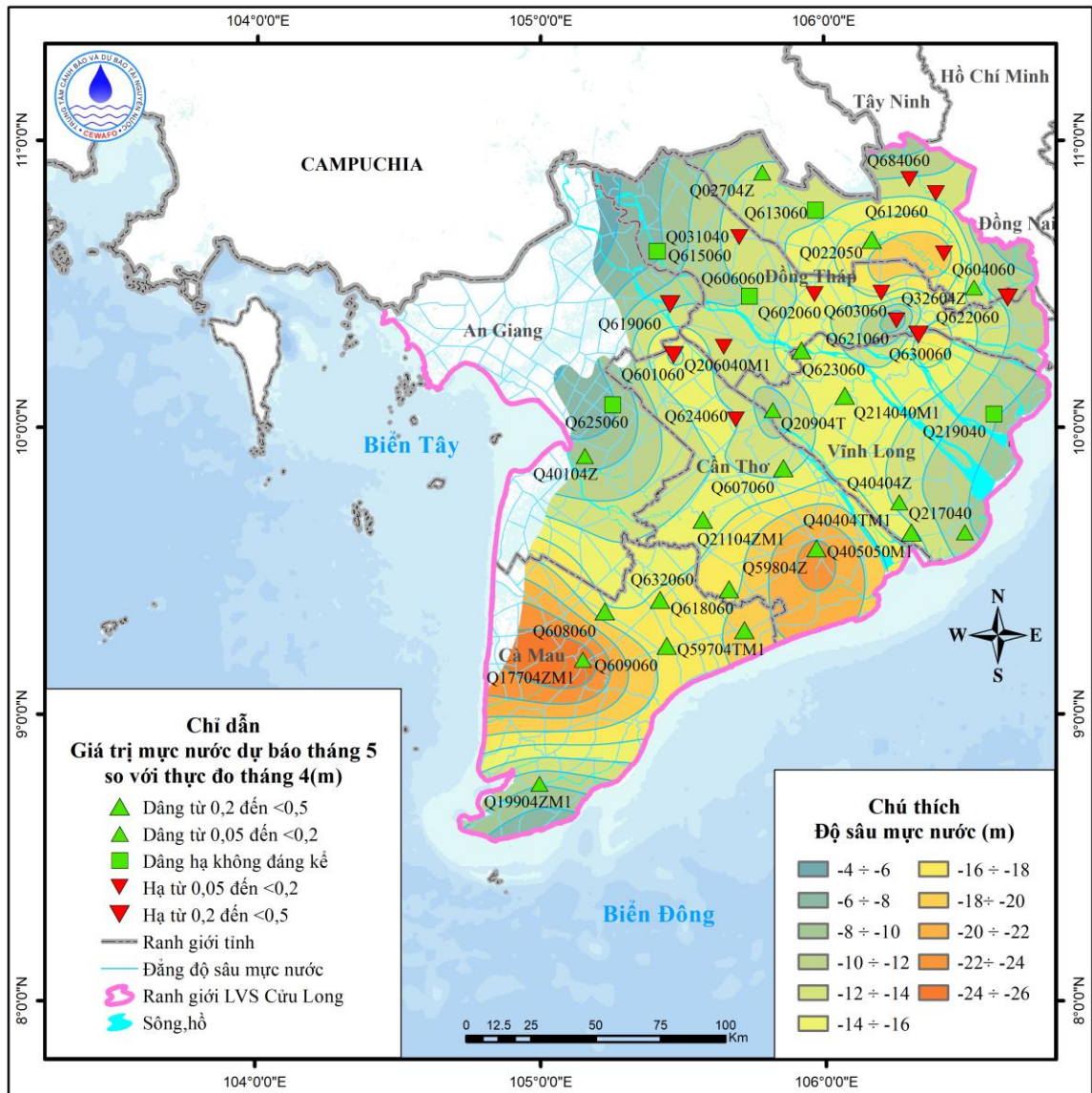
Hình 32. Sơ đồ dự báo diễn biến mực nước tầng n_2^1 tháng 5 năm 2026
