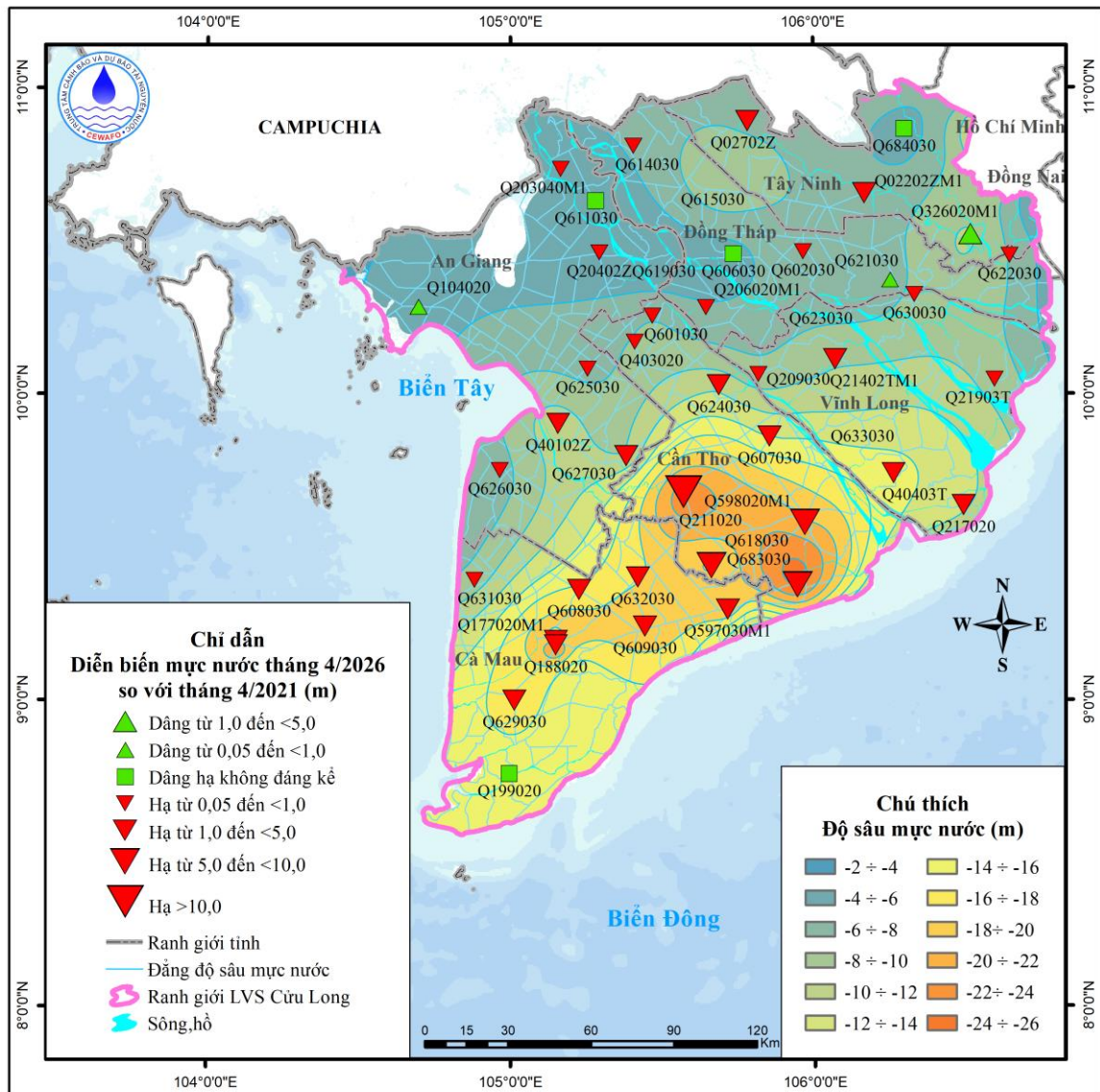
Hình 11. Sơ đồ diễn biến mực nước tháng 4 so với cùng kỳ 5 năm trước d) Tầng chứa nước lỗ hổng trong trầm tích Pleistocene dưới ( qp_1 )
