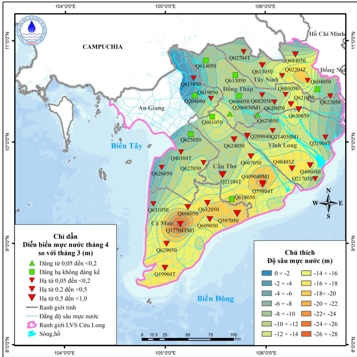
Hình 15. Sơ đồ diễn biến mực nước tháng 4 tầng n_2^2
