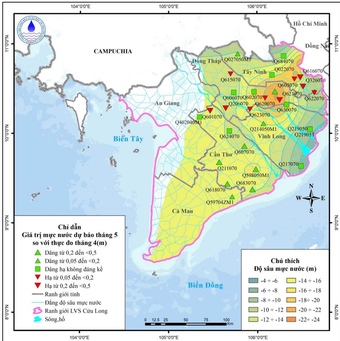
Hình 33. Sơ đồ dự báo diễn biến mực nước tầng n_1^3 tháng 5 năm 2026
