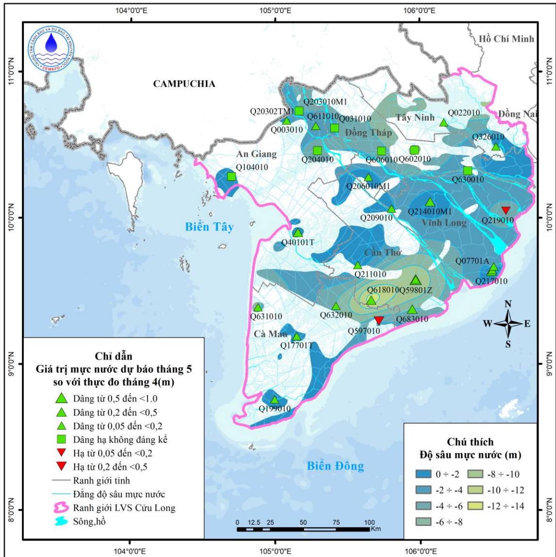
Hình 27. Sơ đồ dự báo diễn biến mực nước tầng qh tháng 5 năm 2026
