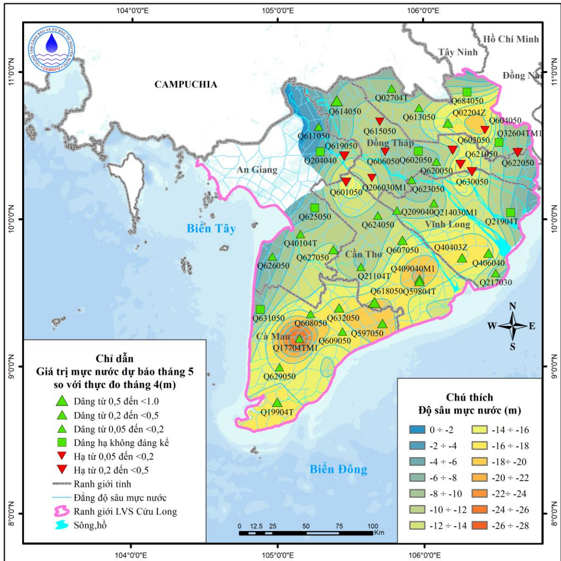
Hình 31. Sơ đồ dự báo diễn biến mực nước tầng n_2^2 tháng 5 năm 2026
