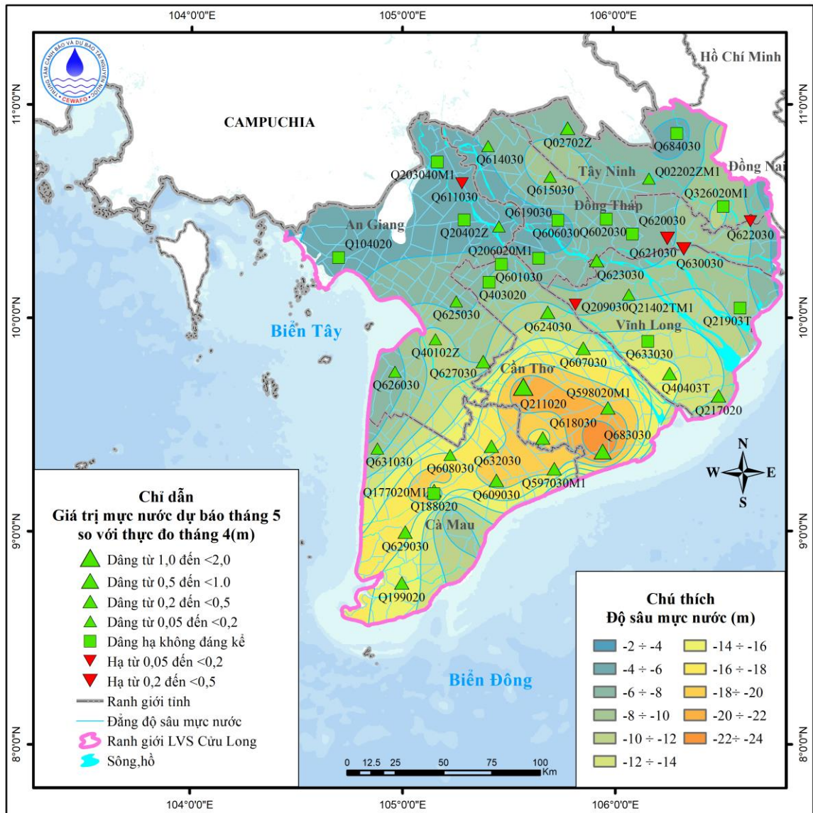
Hình 29. Sơ đồ dự báo diễn biến mực nước tầng qp_{2-3} tháng 5 năm 2026
