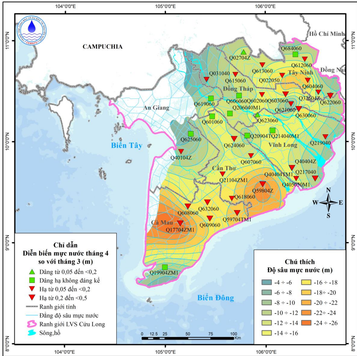
Hình 18. Sơ đồ diễn biến mực nước tháng 4 tầng n_2^1
