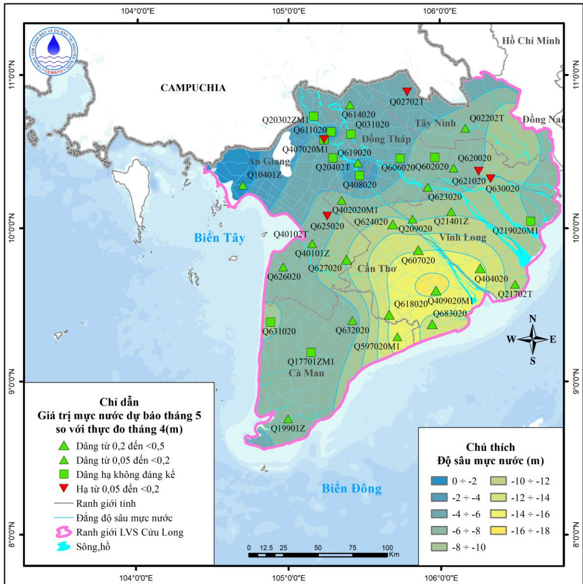
Hình 28. Sơ đồ dự báo diễn biến mực nước tầng qp_3 tháng 5 năm 2026
