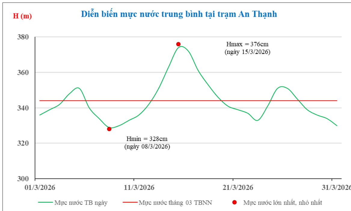
Hình 1. Diễn biến mực nước trung bình ngày tháng 3 năm 2026 tại trạm An Thạnh
