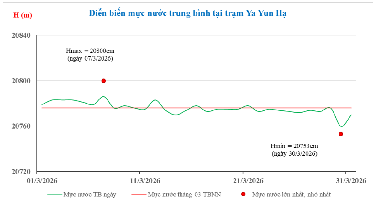
Hình 2. Diễn biến mức nước trung bình ngày tháng 3 năm 2026 tại trạm Ya Yun Hạ
