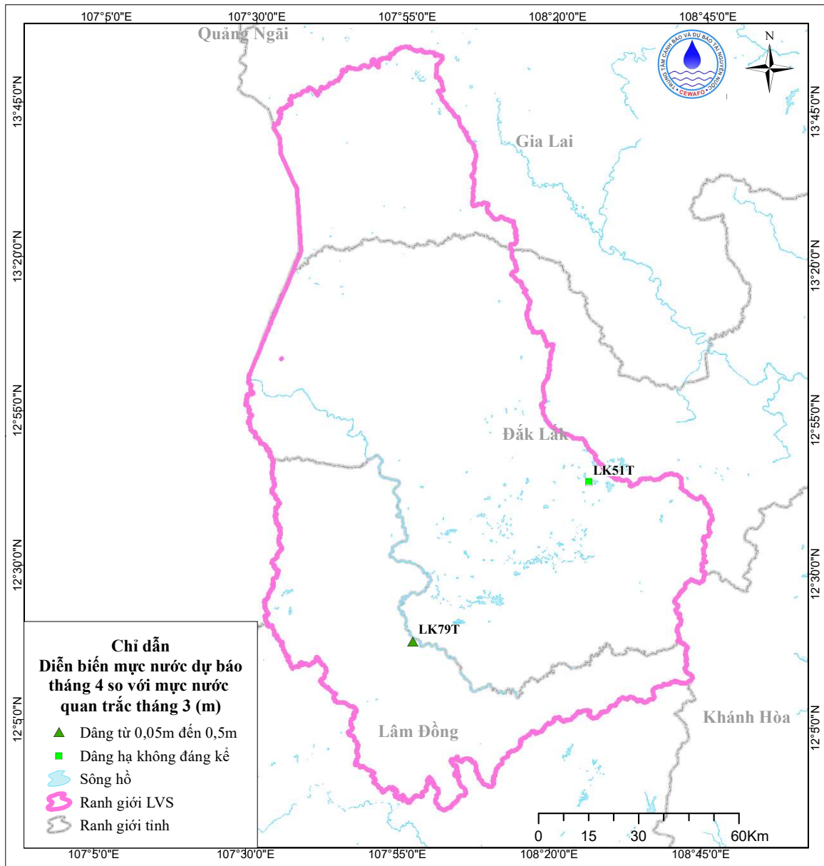
Hình 17. Sơ đồ dự báo diễn biến mực nước tháng 4 tầng q
