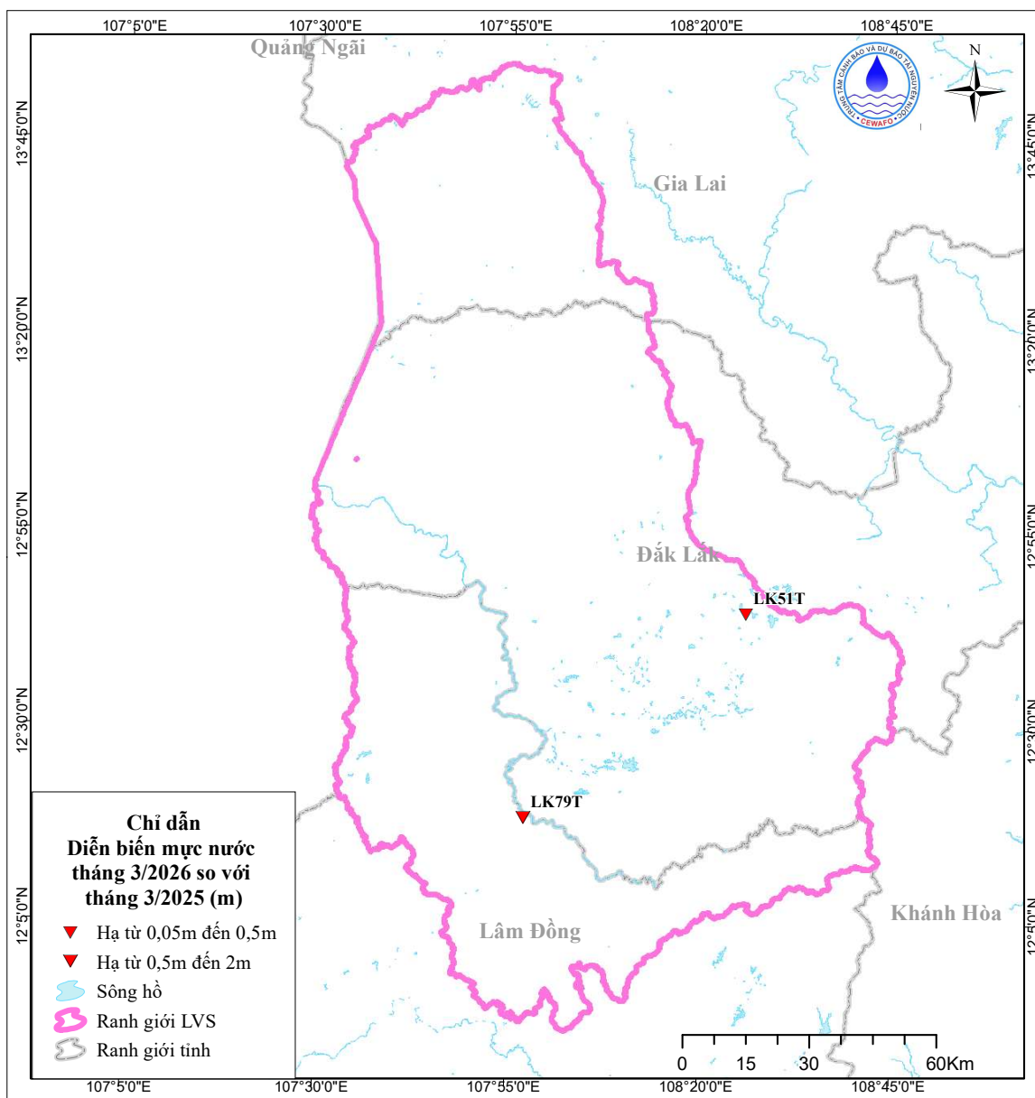
Hình 3. Sơ đồ mực nước trung bình tháng 3 so với cùng kỳ năm trước
