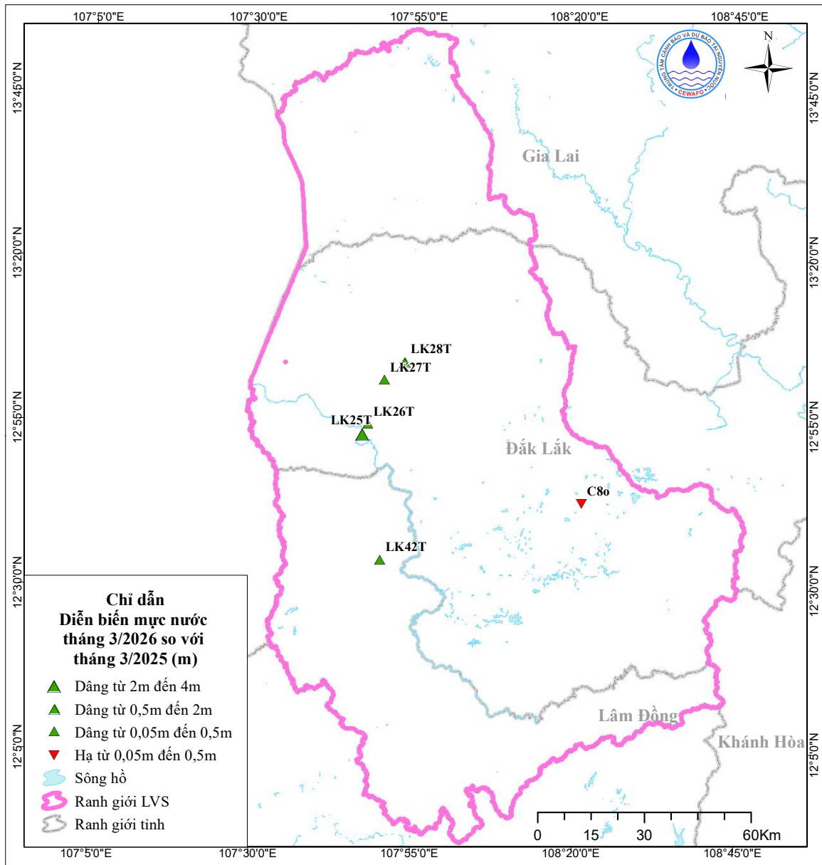
Hình 12. Sơ đồ mực nước trung bình tháng 3 so với cùng kỳ năm trước
