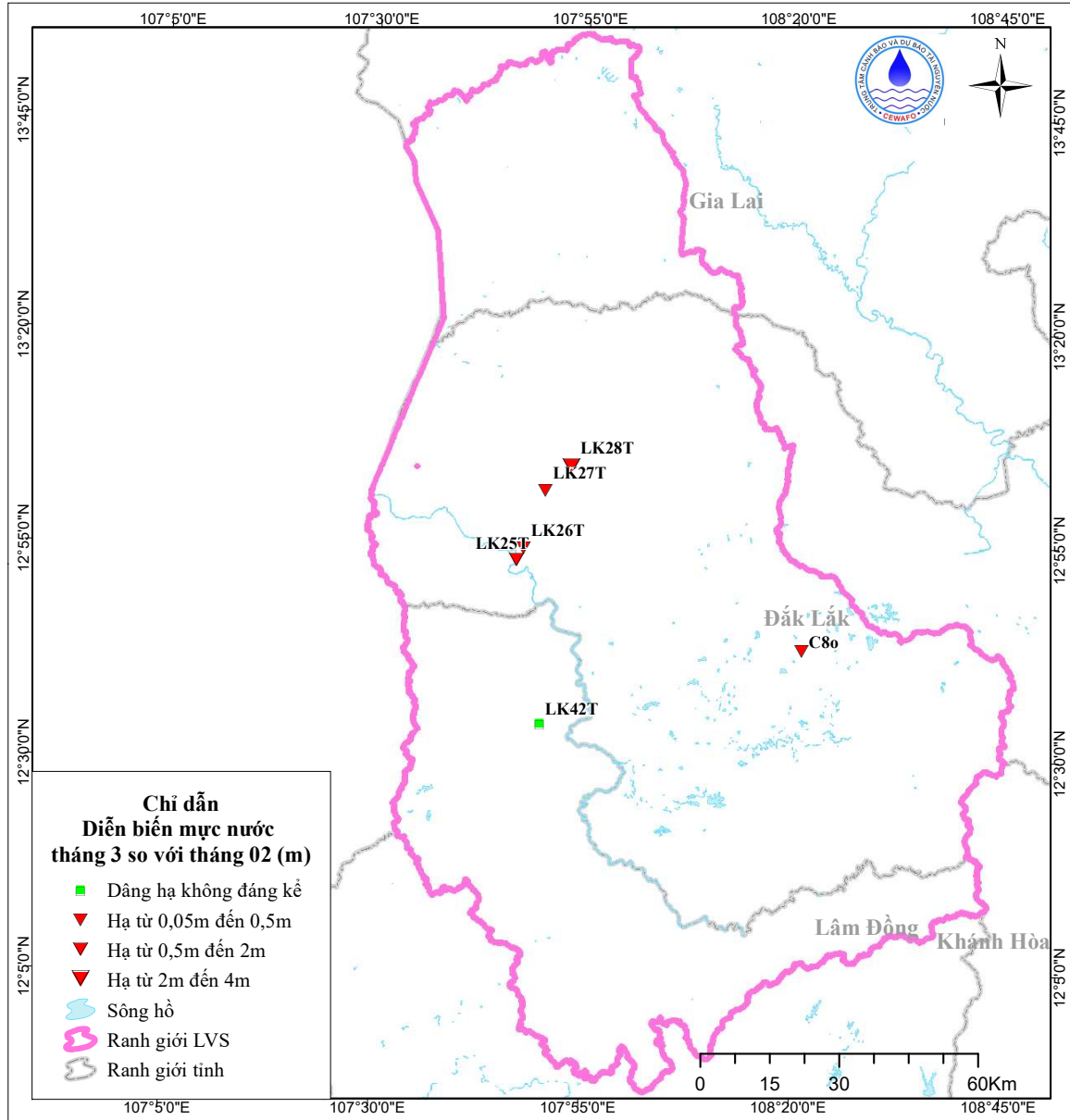
Hình 11. Sơ đồ diễn biến mực nước tháng 3 tầng j_{1-2}
