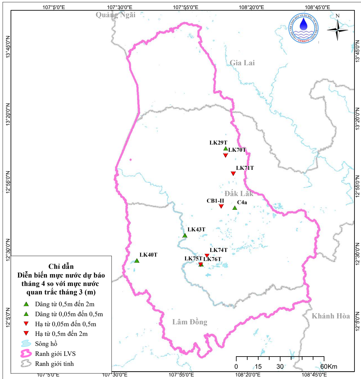
Hình 18. Sơ đồ dự báo diễn biến mực nước tháng 4 tầng \beta(qp)
