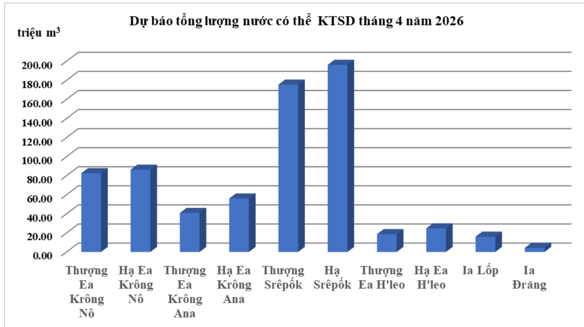
Hình 16. Biểu đồ dự báo lượng nước có thể KTSD tháng 4 năm 2026
