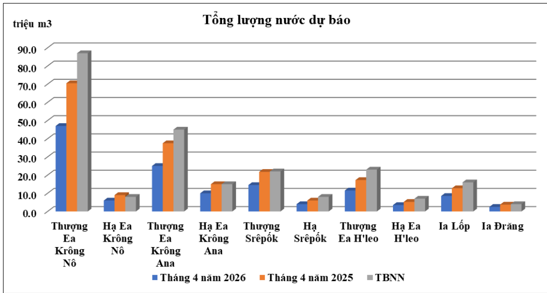
Hình 14. Biểu đồ tổng lượng nước dự báo tháng 4 năm 2026
