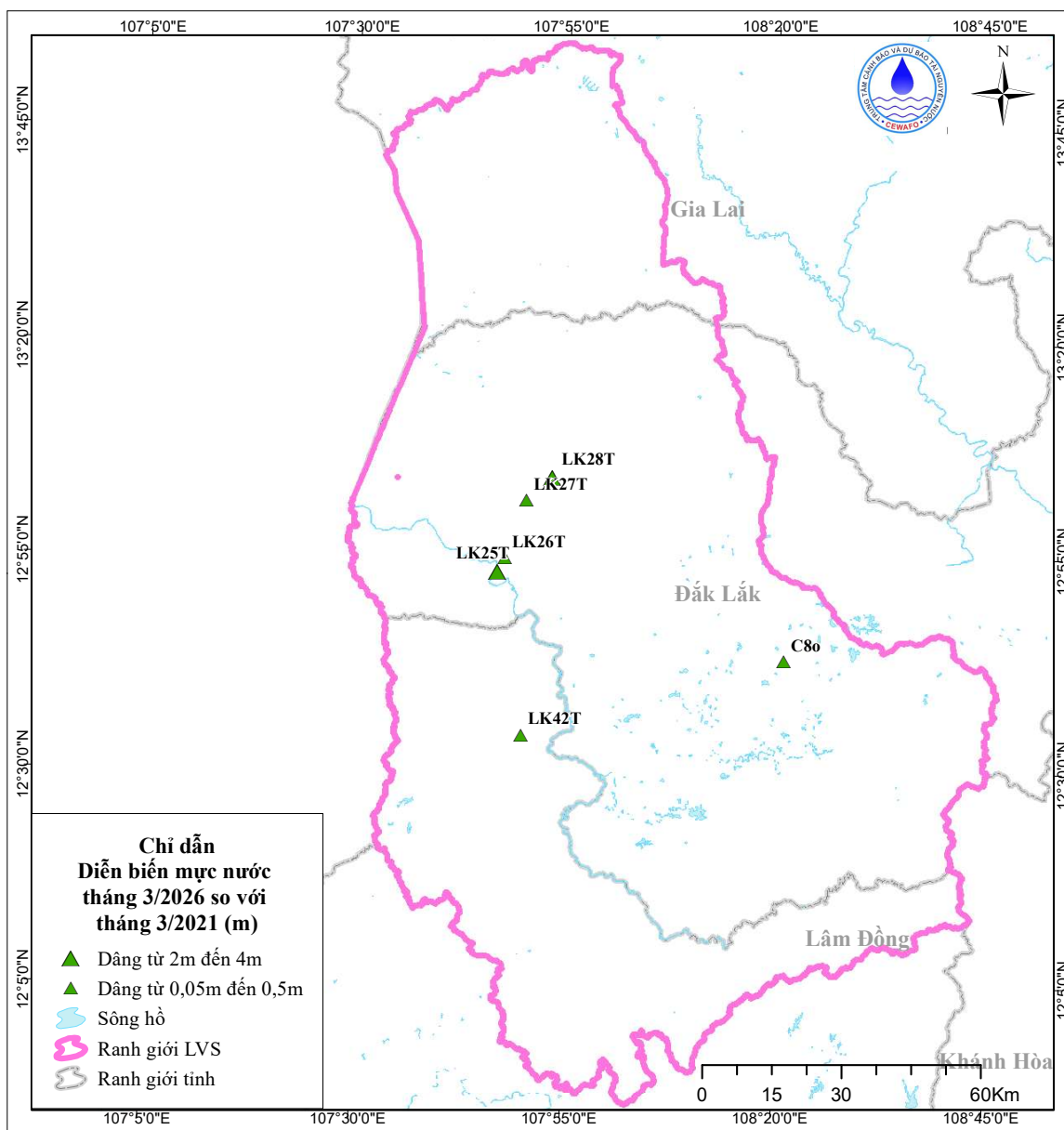
Hình 13. Sơ đồ mực nước trung bình tháng 3 so với cùng kỳ 5 năm trước
