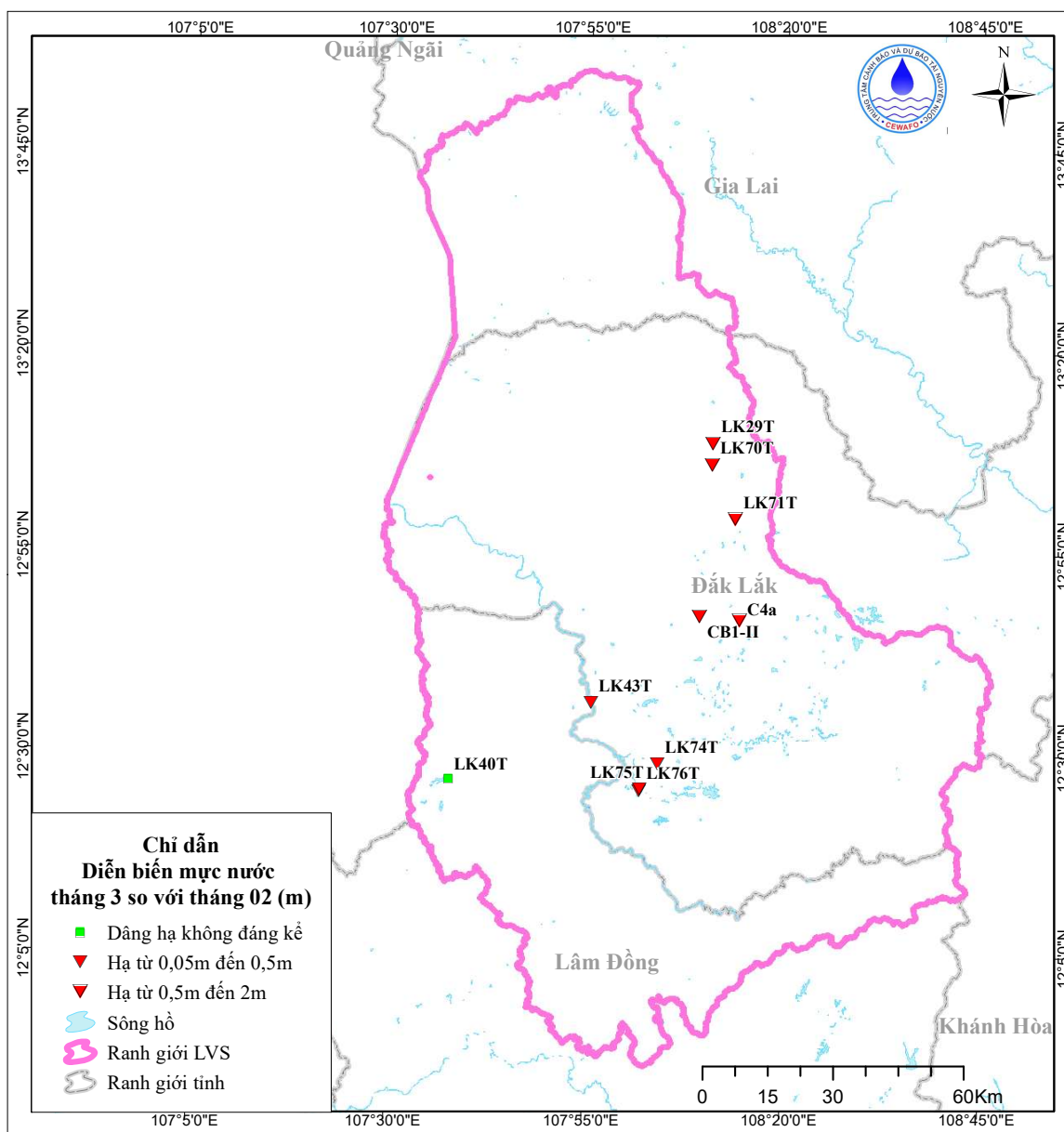
Hình 5. Sơ đồ diễn biến mực nước tháng 3 tầng \beta (qp)
