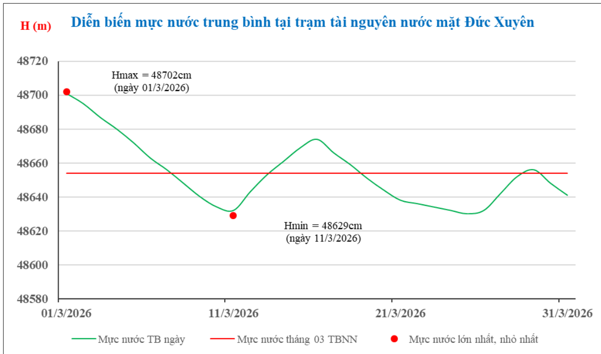
Hình 1. Diễn biến mực nước trung bình ngày tháng 3 năm 2026 tại trạm tài nguyên nước mặt Đức Xuyên
