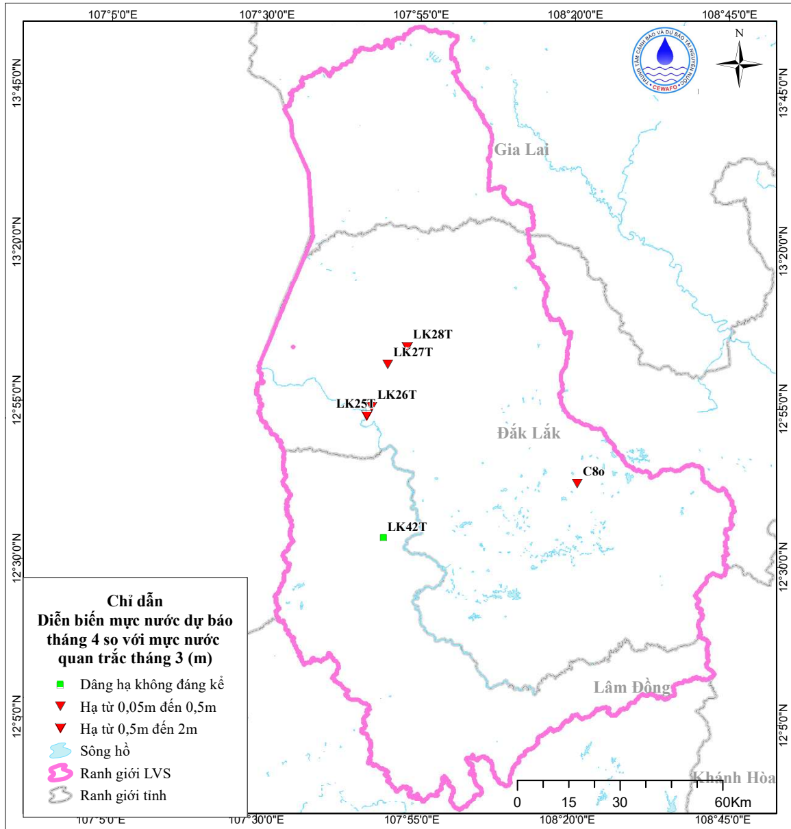
Hình 20. Sơ đồ dự báo diễn biến mực nước tháng 4 tầng (j 1-2 )
