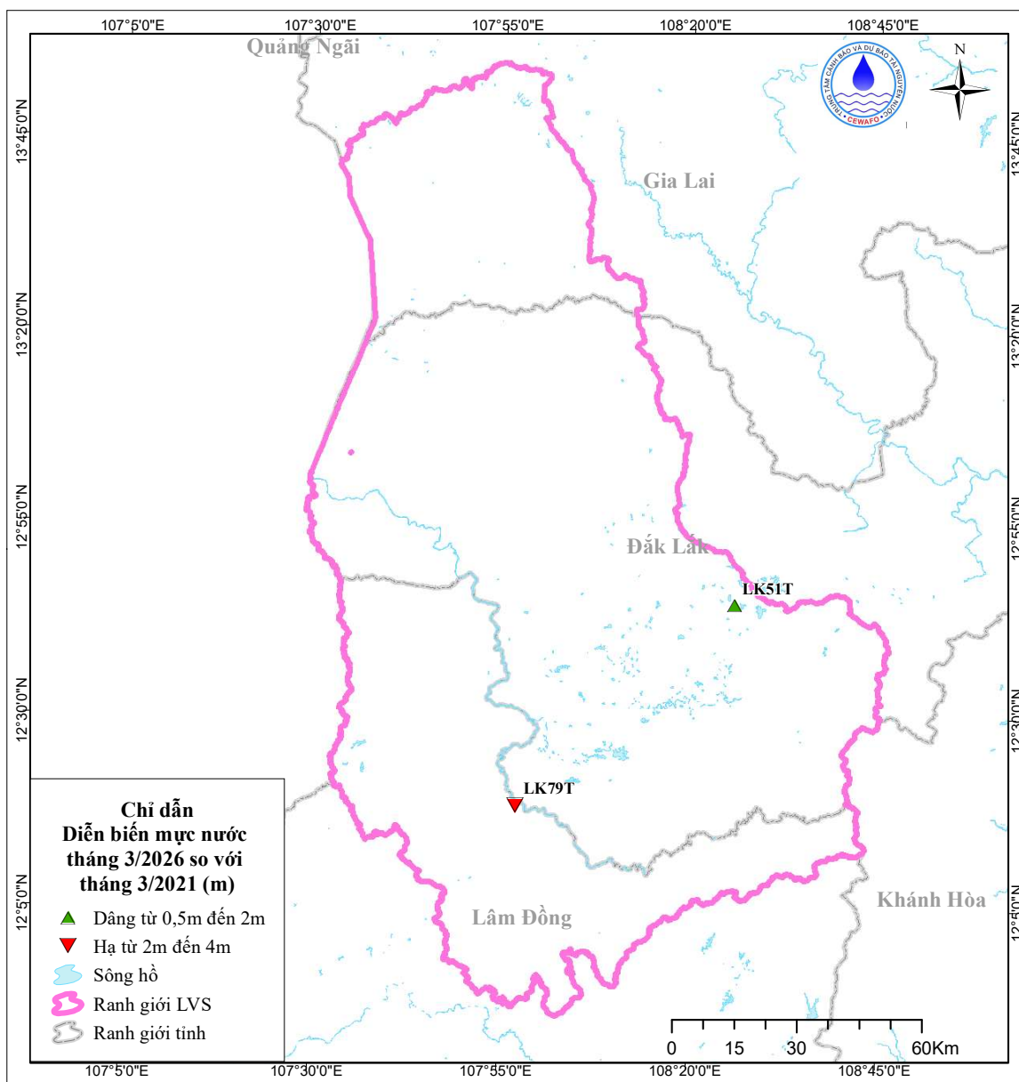
Hình 4. Sơ đồ mực nước trung bình tháng 3 so với cùng kỳ 5 năm trước
