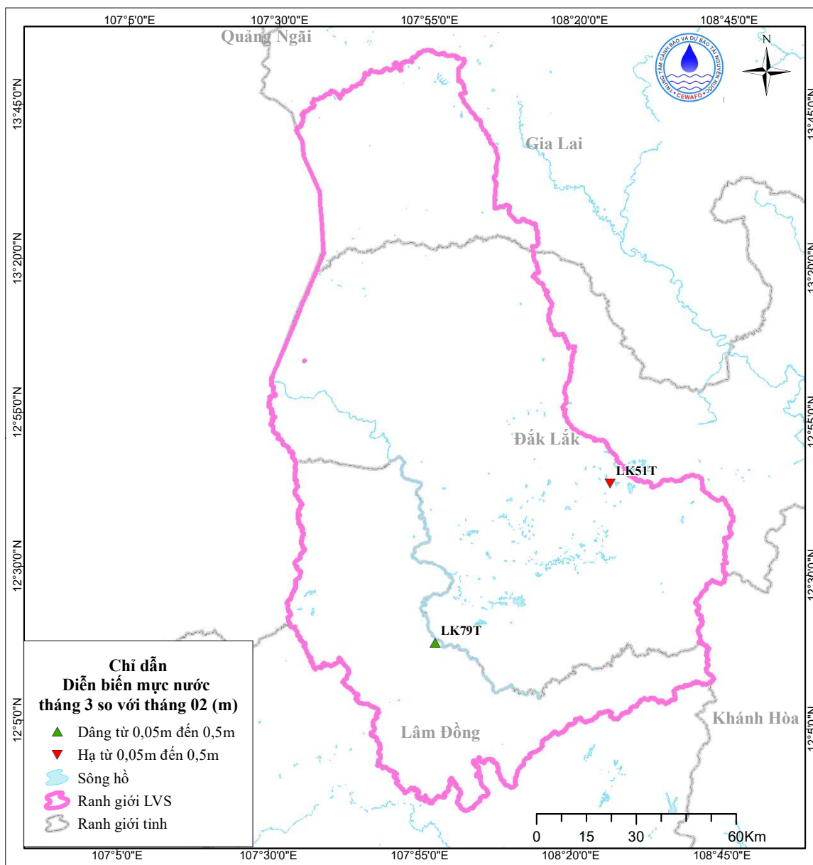
Hình 2. Sơ đồ diễn biến mực nước tháng 3 tầng q
