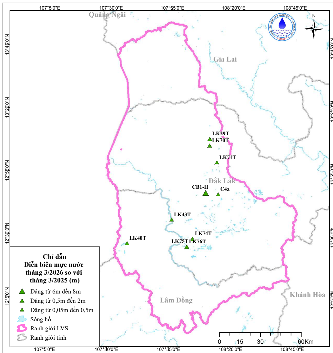
Hình 6. Sơ đồ mực nước trung bình tháng 3 so với cùng kỳ năm trước
