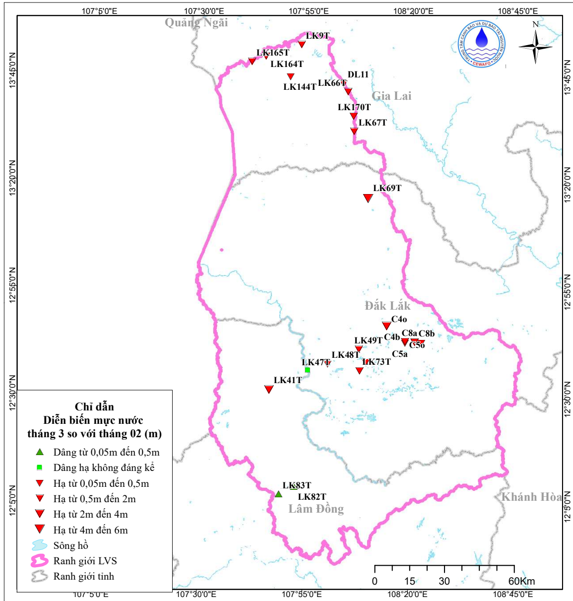
Hình 8. Sơ đồ diễn biến mực nước tháng 3 tầng \beta(n_2-qp)
