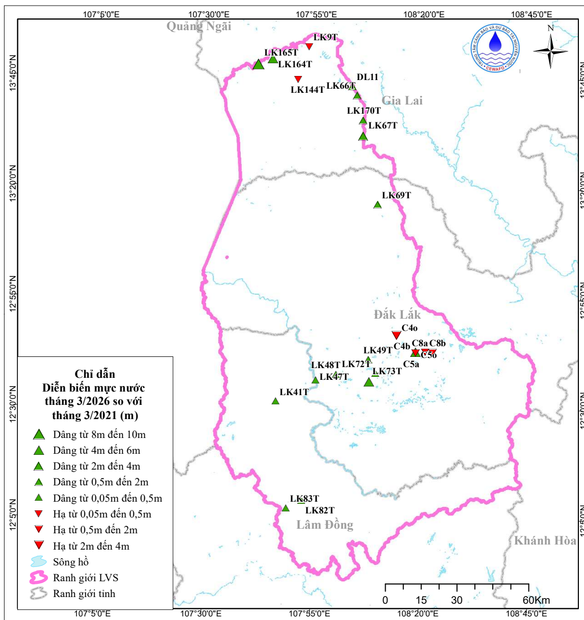
Hình 10. Sơ đồ mực nước trung bình tháng 3 so với cùng kỳ 5 năm trước
