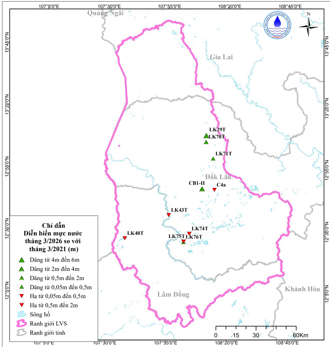
Hình 7. Sơ đồ mực nước trung bình tháng 3 so với cùng kỳ 5 năm trước
