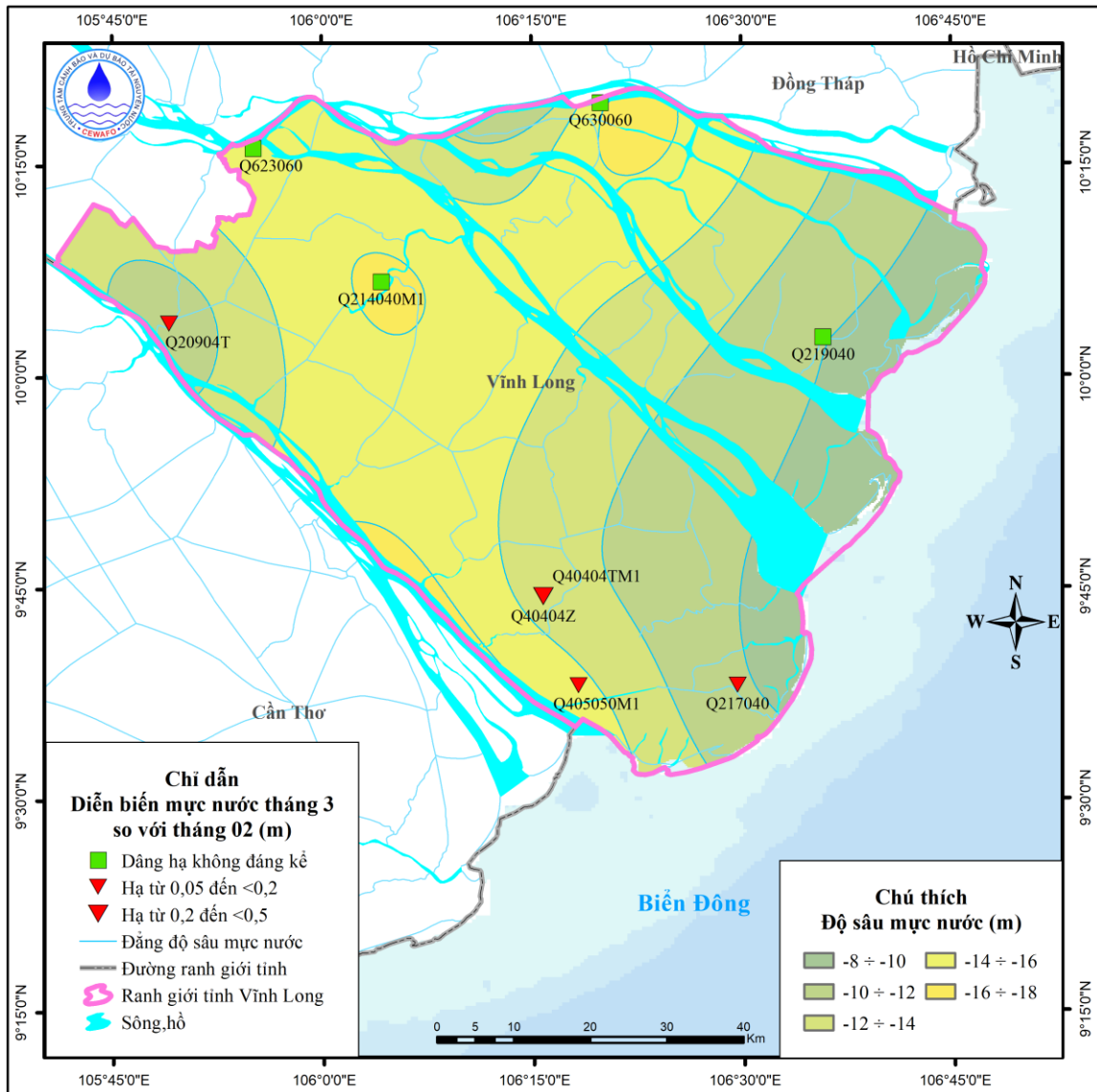
Hình 6. Sơ đồ diễn biến mực nước tháng 3 tầng n_2^1 g) Tầng chứa nước lỗ hổng trong các đá trầm tích Miocene trên ( n_1^3 )
