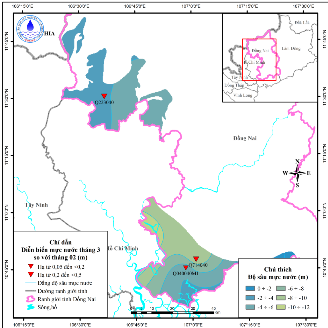
Hình 3. Sơ đồ diễn biến mực nước tháng 3 tầng n_2^2
