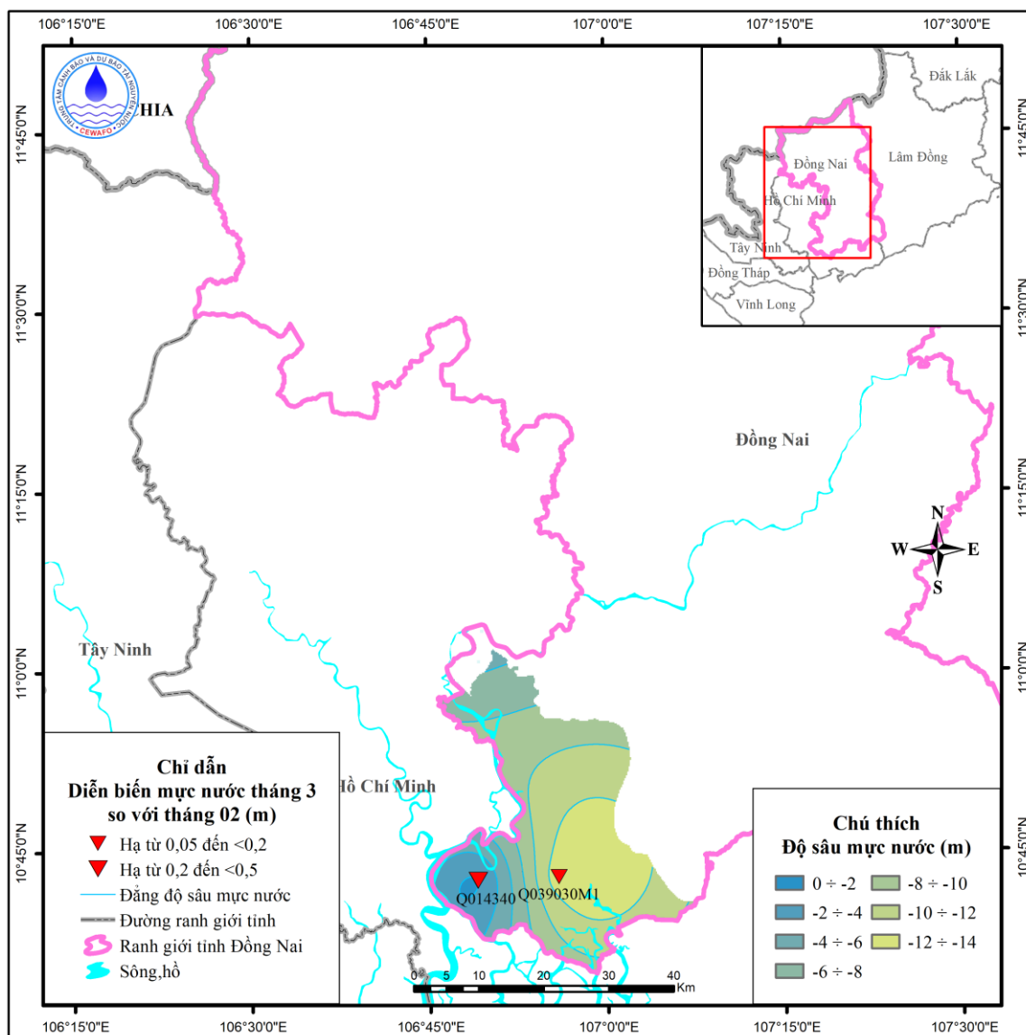
Hình 1. Sơ đồ diễn biến mực nước tháng 3 tầng qp_{2-3}
