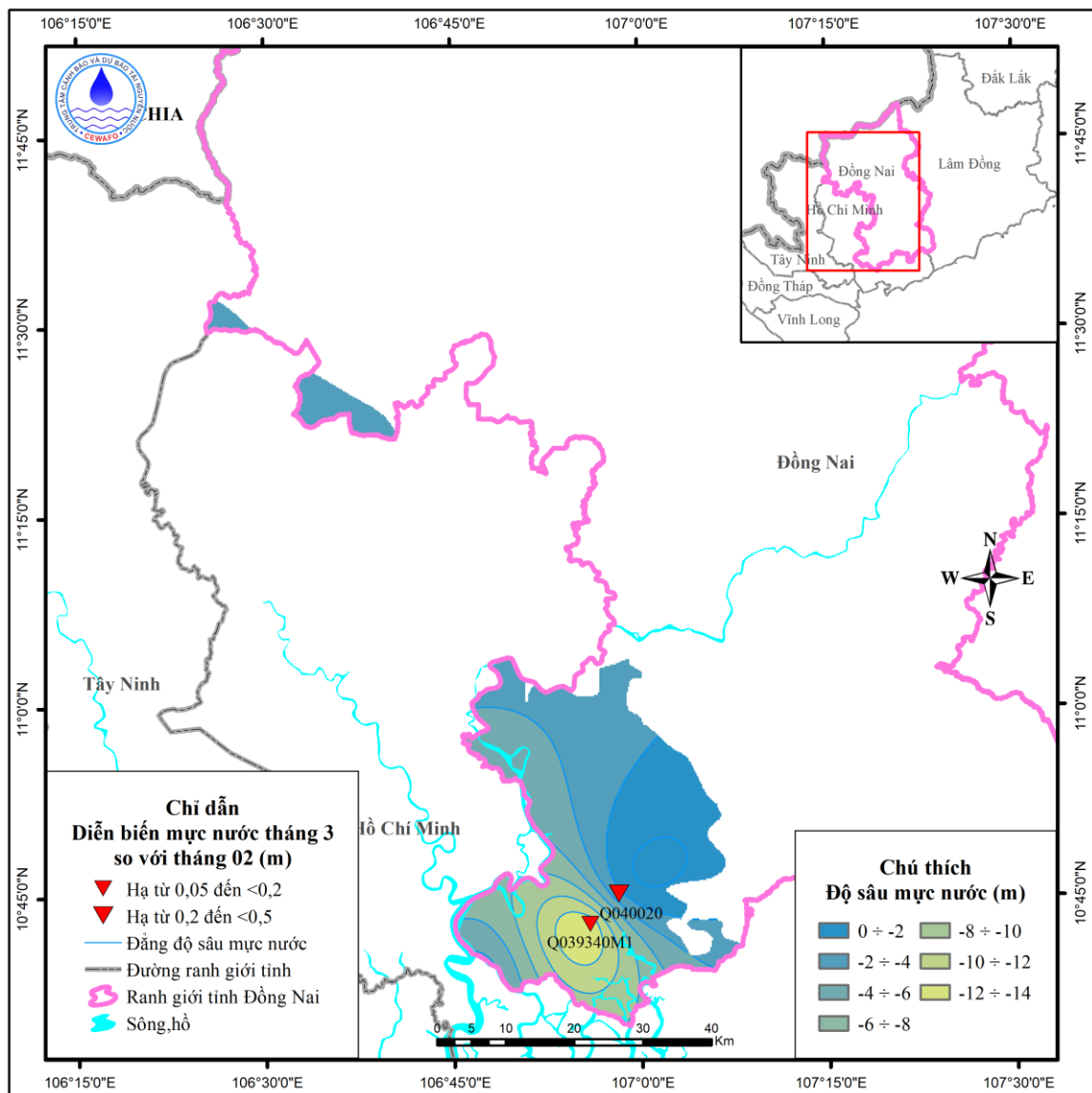
Hình 2. Sơ đồ diễn biến mực nước tháng 3 tầng q_1
