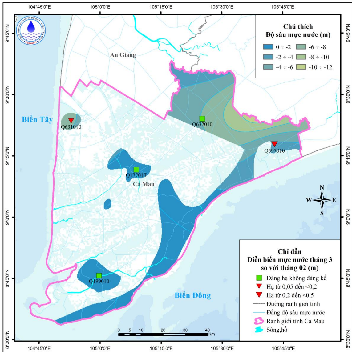
Hình 1. Sơ đồ diễn biến mực nước tháng 3 tầng qh b) Tầng chứa nước lỗ hổng trong trầm tích Pleistocene trên (qp 3 )
