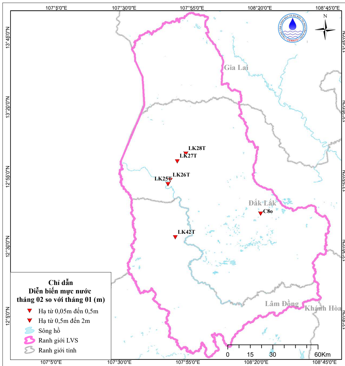
Hình 11. Sơ đồ diễn biến mực nước tháng 02 tầng j_{1-2}
