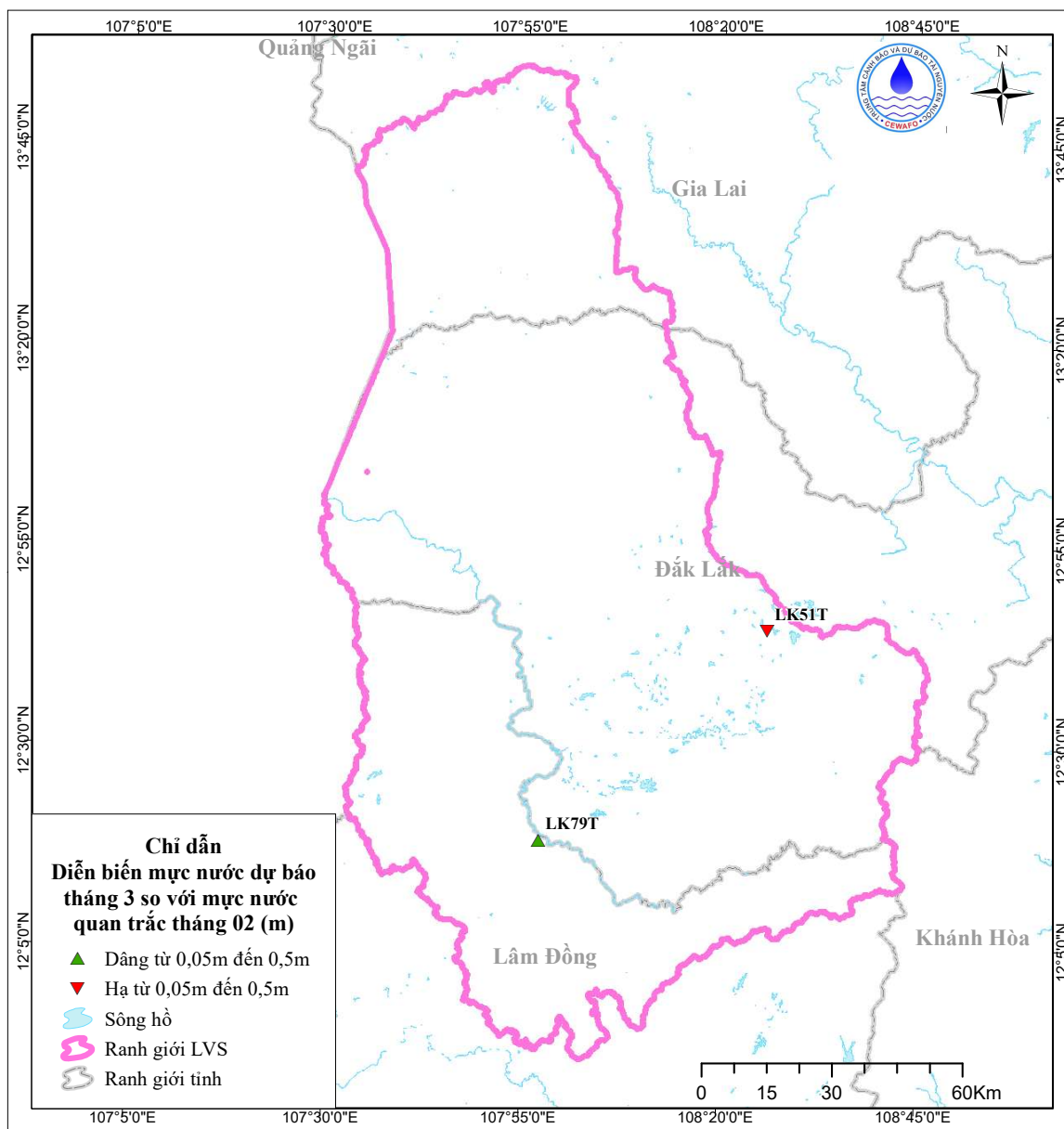
Hình 17. Sơ đồ dự báo diễn biến mực nước tháng 3 tầng q
