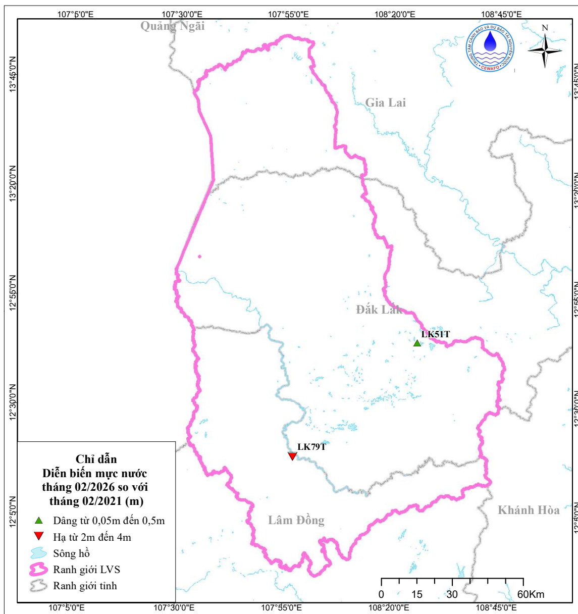
Hình 4. Sơ đồ mực nước trung bình tháng 02 so với cùng kỳ 5 năm trước
