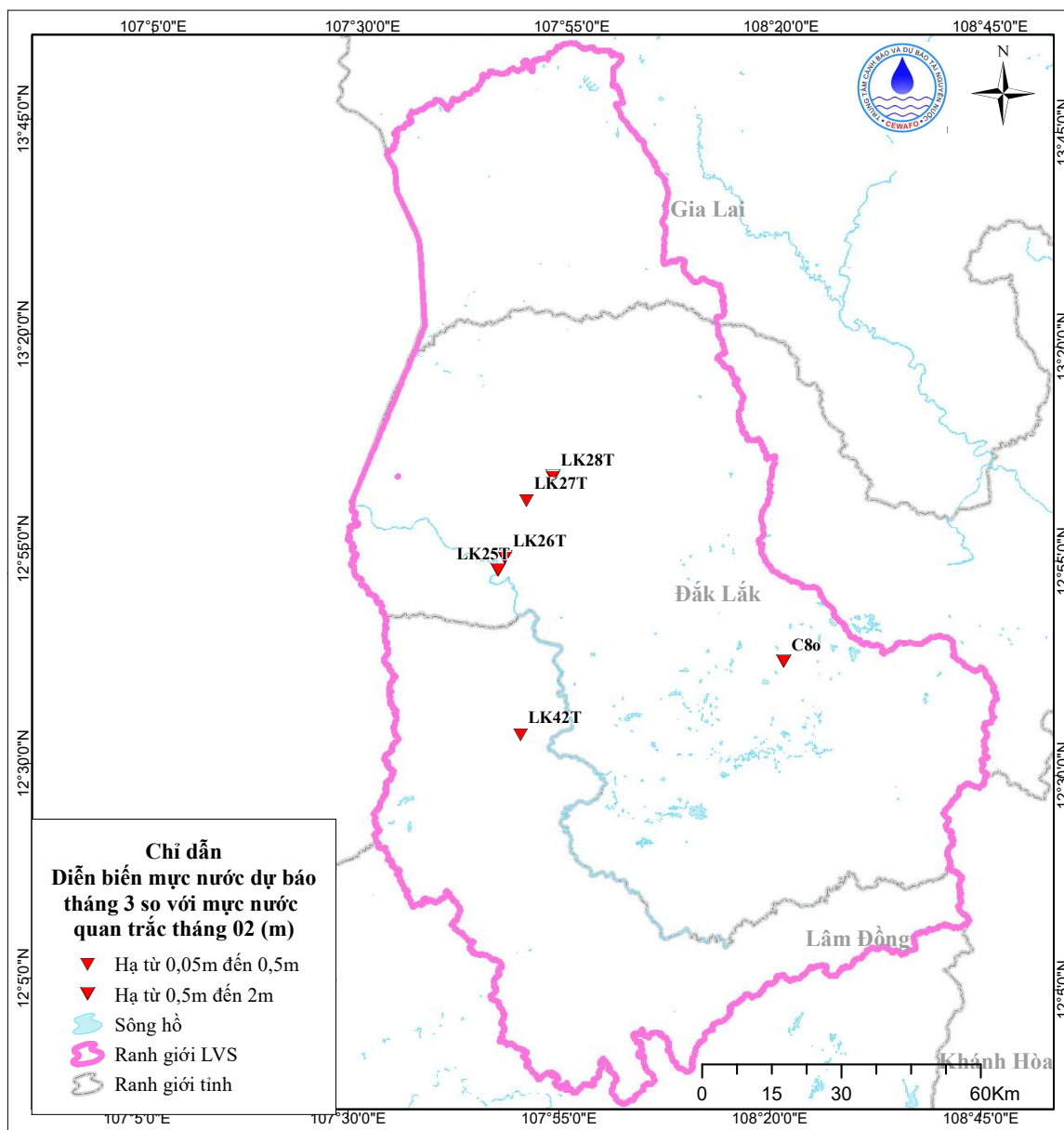
Hình 20. Sơ đồ dự báo diễn biến mực nước tháng 3 tầng (j 1-2 )
