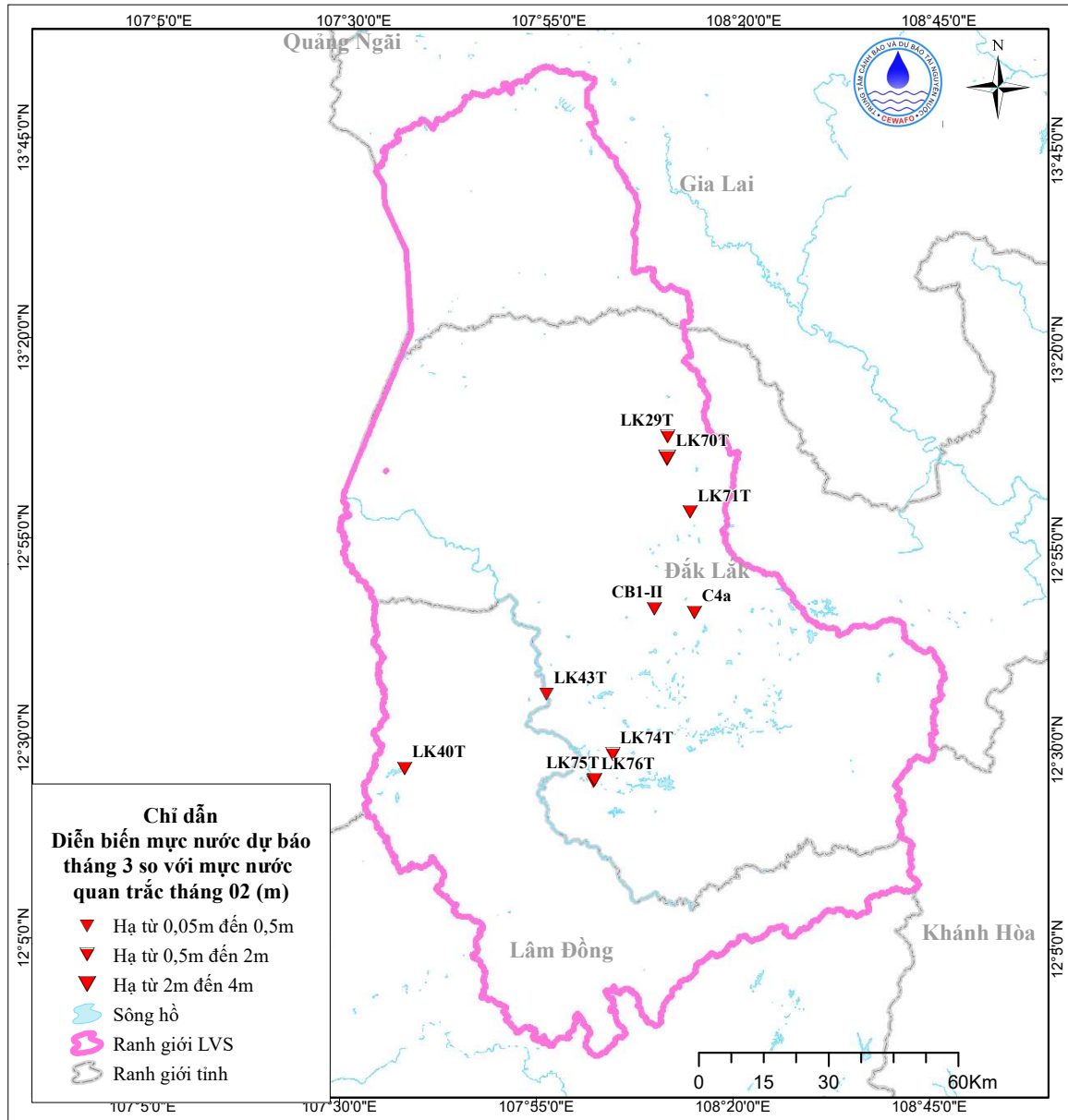
Hình 18. Sơ đồ dự báo diễn biến mực nước tháng 3 tầng \beta(qp)
