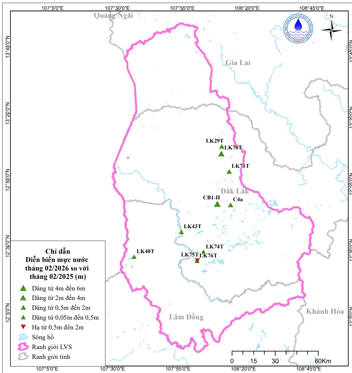
Hình 6. Sơ đồ mực nước trung bình tháng 02 so với cùng kỳ năm trước
