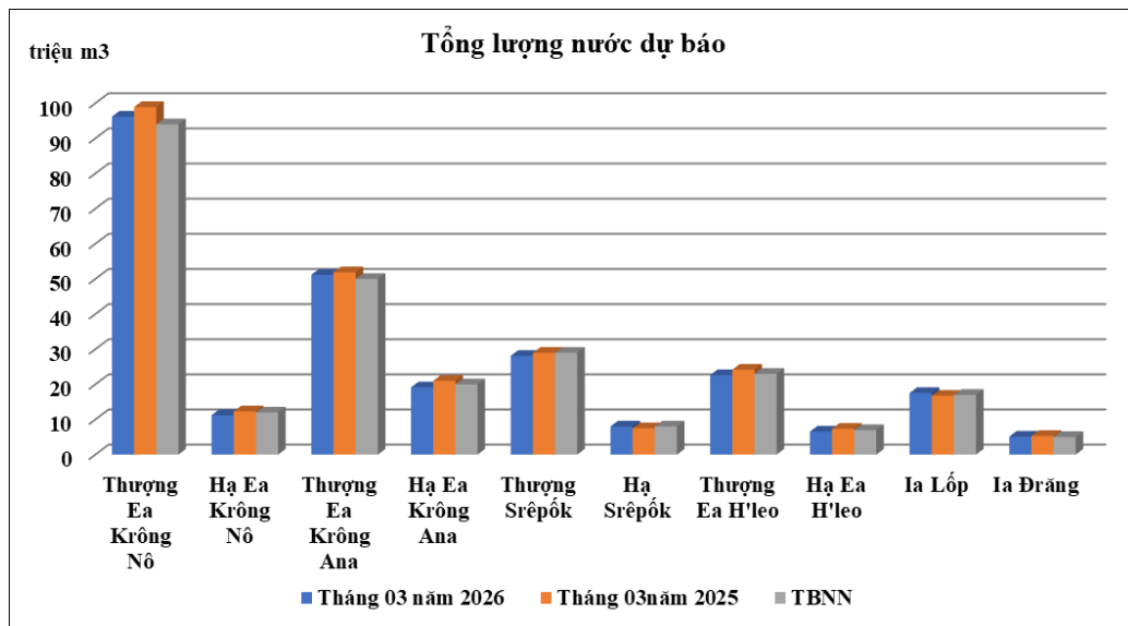
Hình 14. Biểu đồ tổng lượng nước dự báo tháng 3 năm 2026
