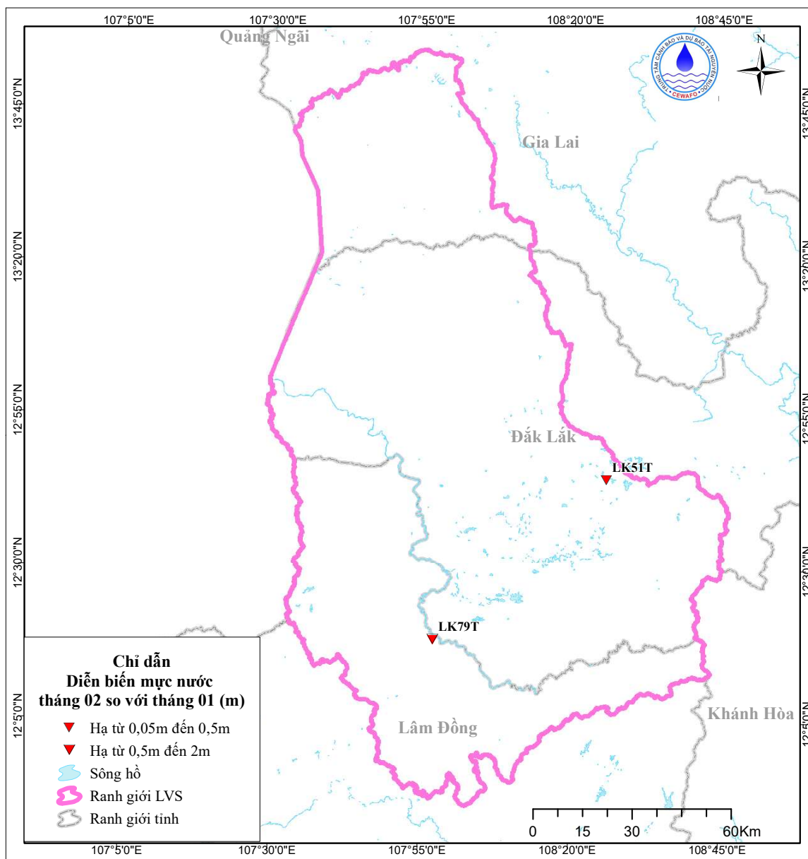
Hình 2. Sơ đồ diễn biến mực nước tháng 02 tăng q
