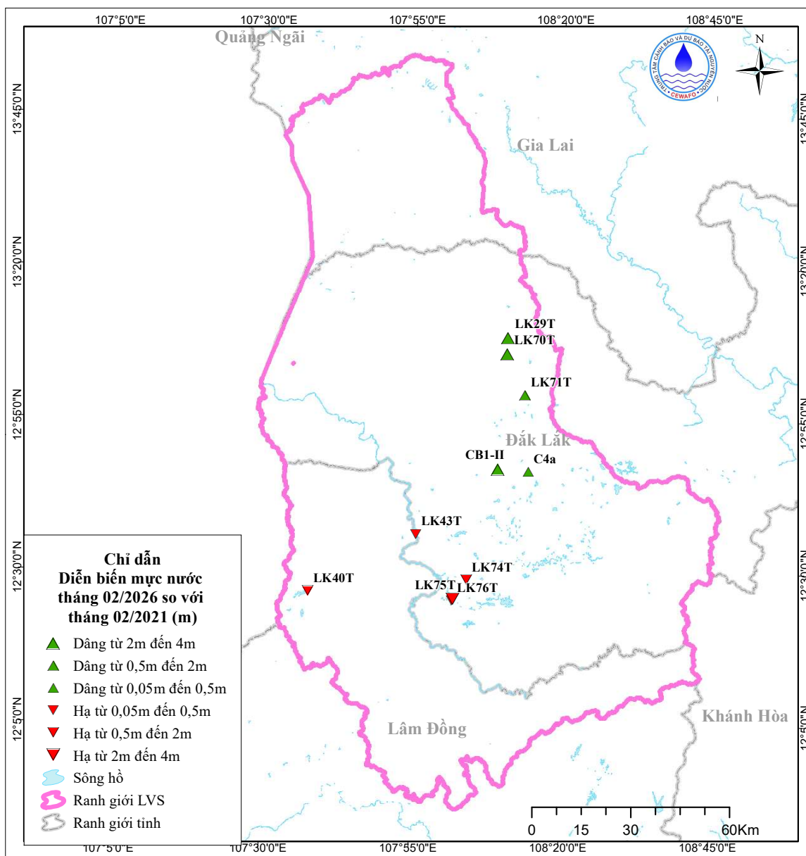
Hình 7. Sơ đồ mực nước trung bình tháng 02 so với cùng kỳ 5 năm trước
