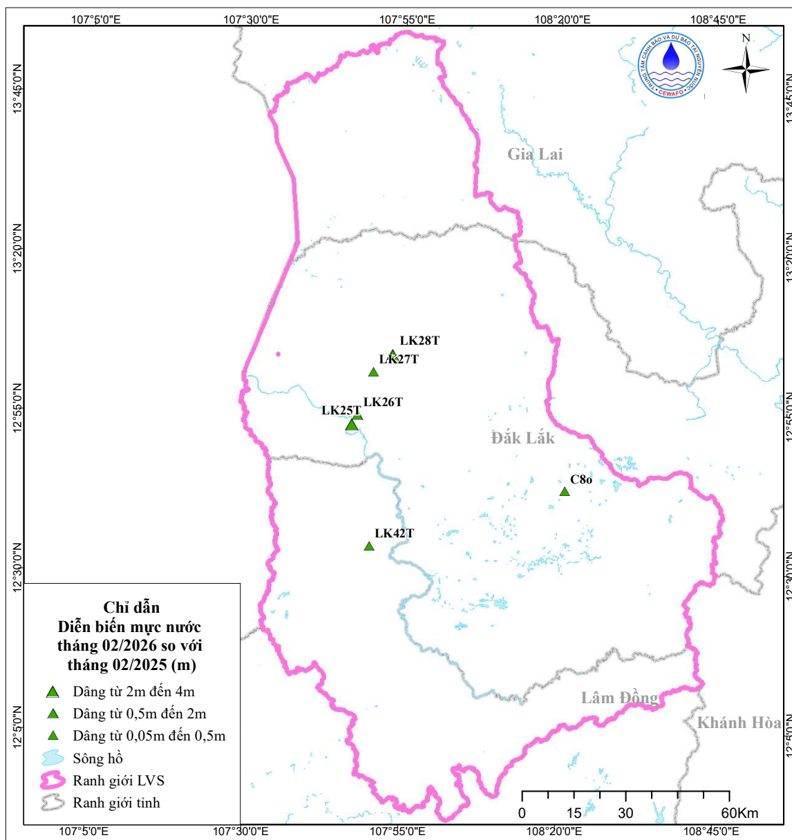
Hình 12. Sơ đồ mực nước trung bình tháng 02 so với cùng kỳ năm trước
