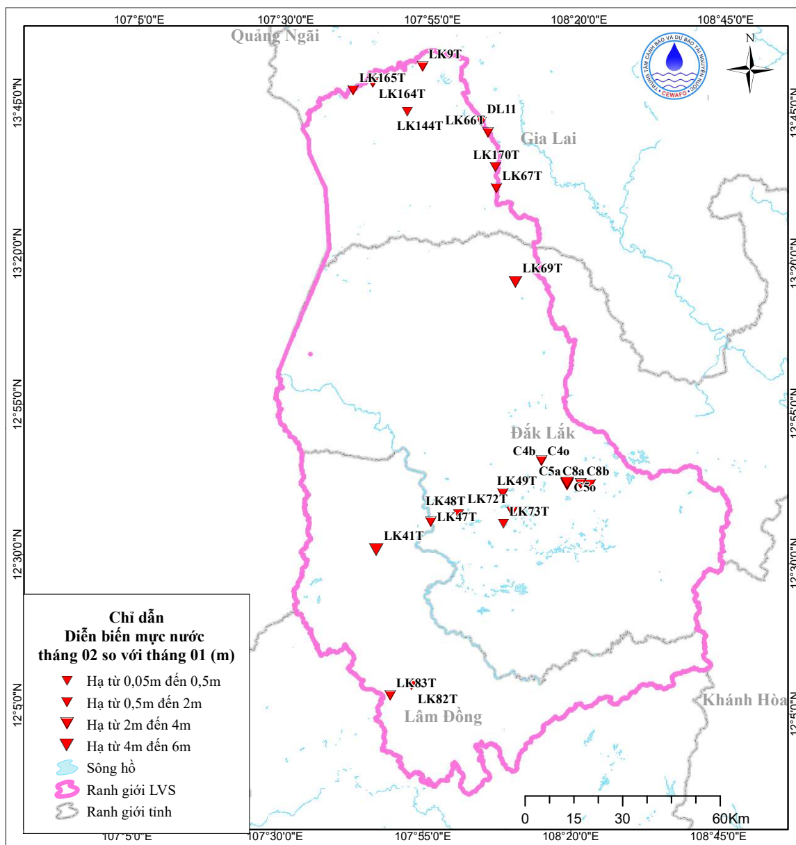
Hình 8. Sơ đồ diễn biến mực nước tháng 02 tầng \beta(n_2-qp)
