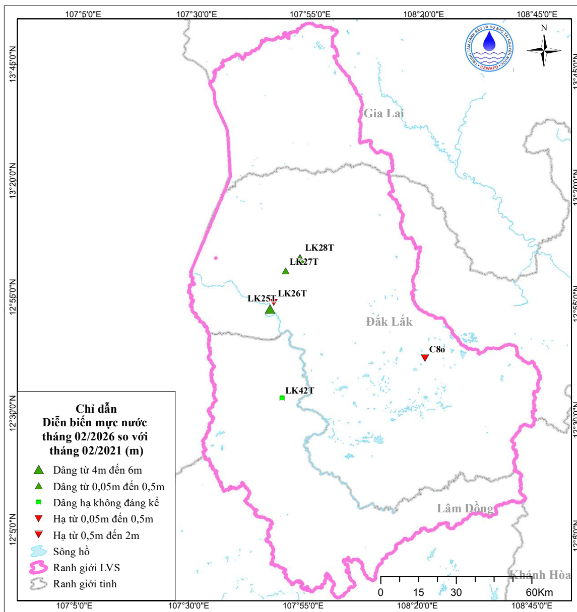
Hình 13. Sơ đồ mực nước trung bình tháng 02 so với cùng kỳ 5 năm trước
