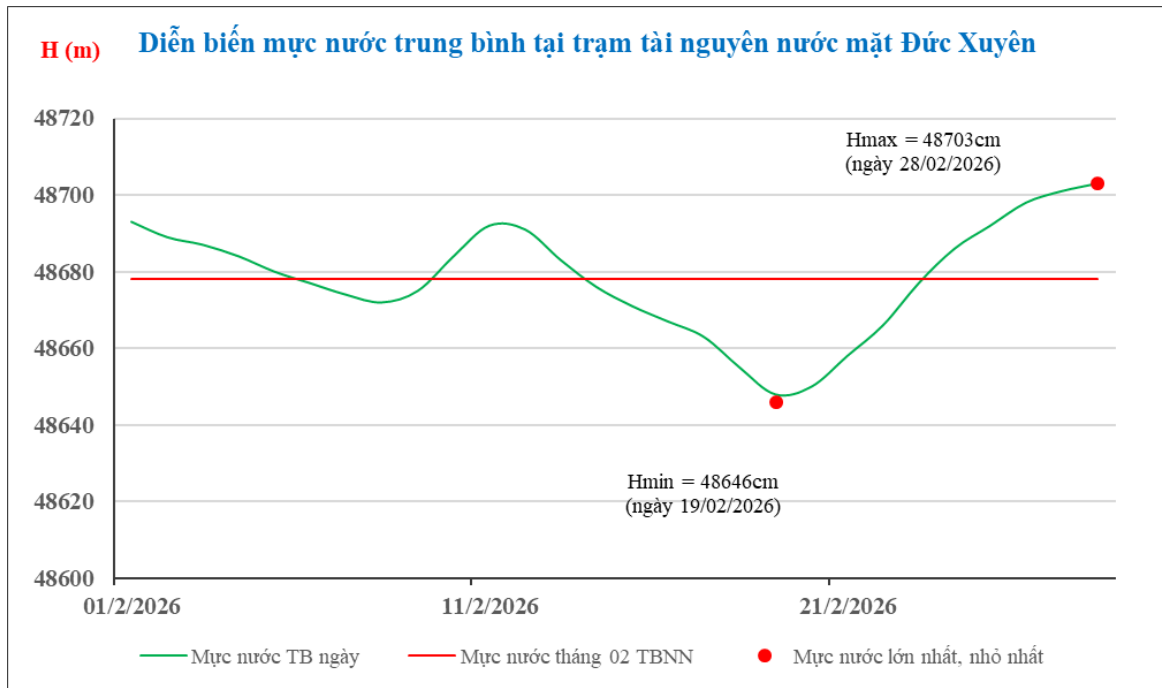
Hình 1. Diễn biến mực nước trung bình ngày tháng 02 năm 2026 tại trạm tài nguyên nước mặt Đức Xuyên
