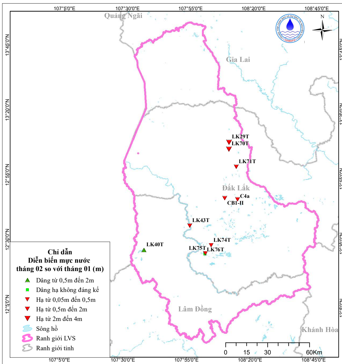
Hình 5. Sơ đồ diễn biến mực nước tháng 02 tầng \beta (qp)
