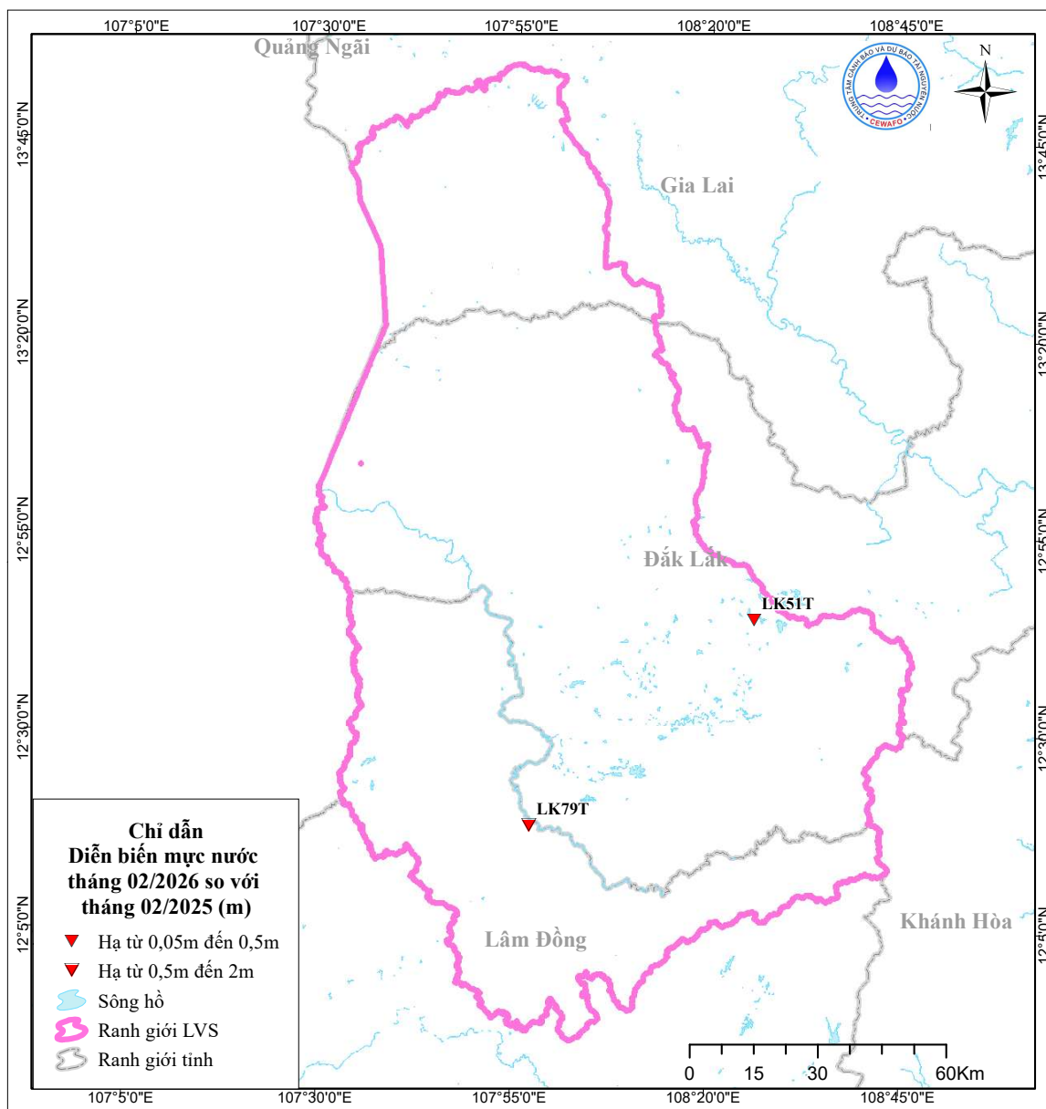
Hình 3. Sơ đồ mực nước trung bình tháng 02 so với cùng kỳ năm trước
