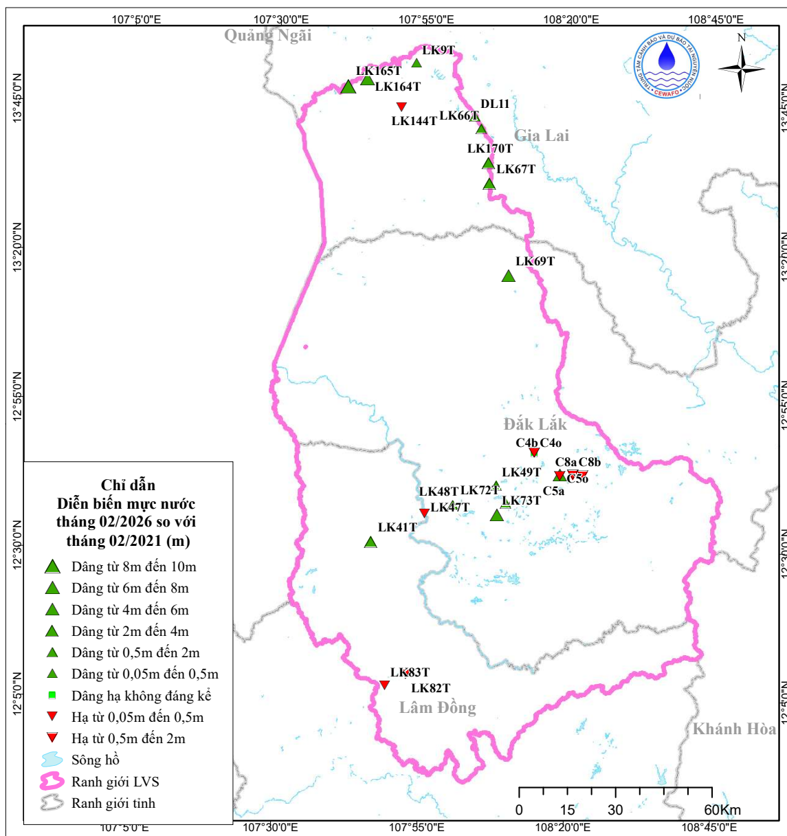
Hình 10. Sơ đồ mực nước trung bình tháng 02 so với cùng kỳ 5 năm trước
