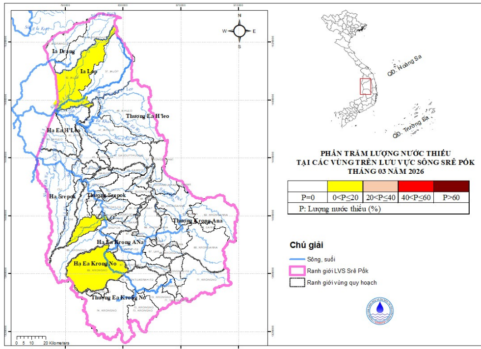
Hình 16. Biểu đồ dự báo lượng nước thiếu tháng 3 năm 2026
