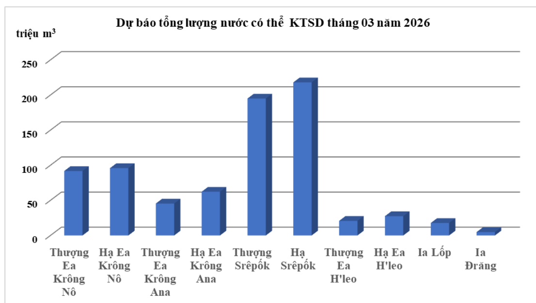
Hình 16. Biểu đồ dự báo lượng nước có thể KTSD tháng 3 năm 2026
