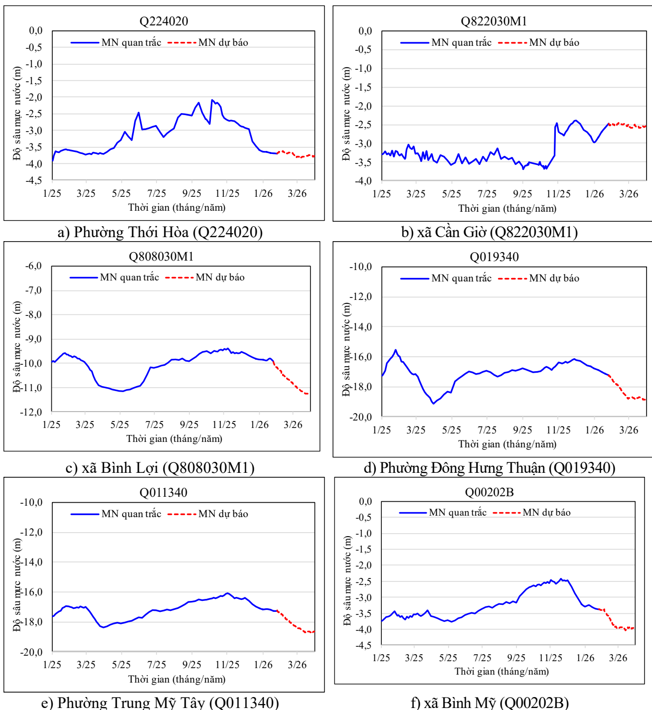
Hình 10. Dự báo độ sâu mực nước tầng qp 2-3
