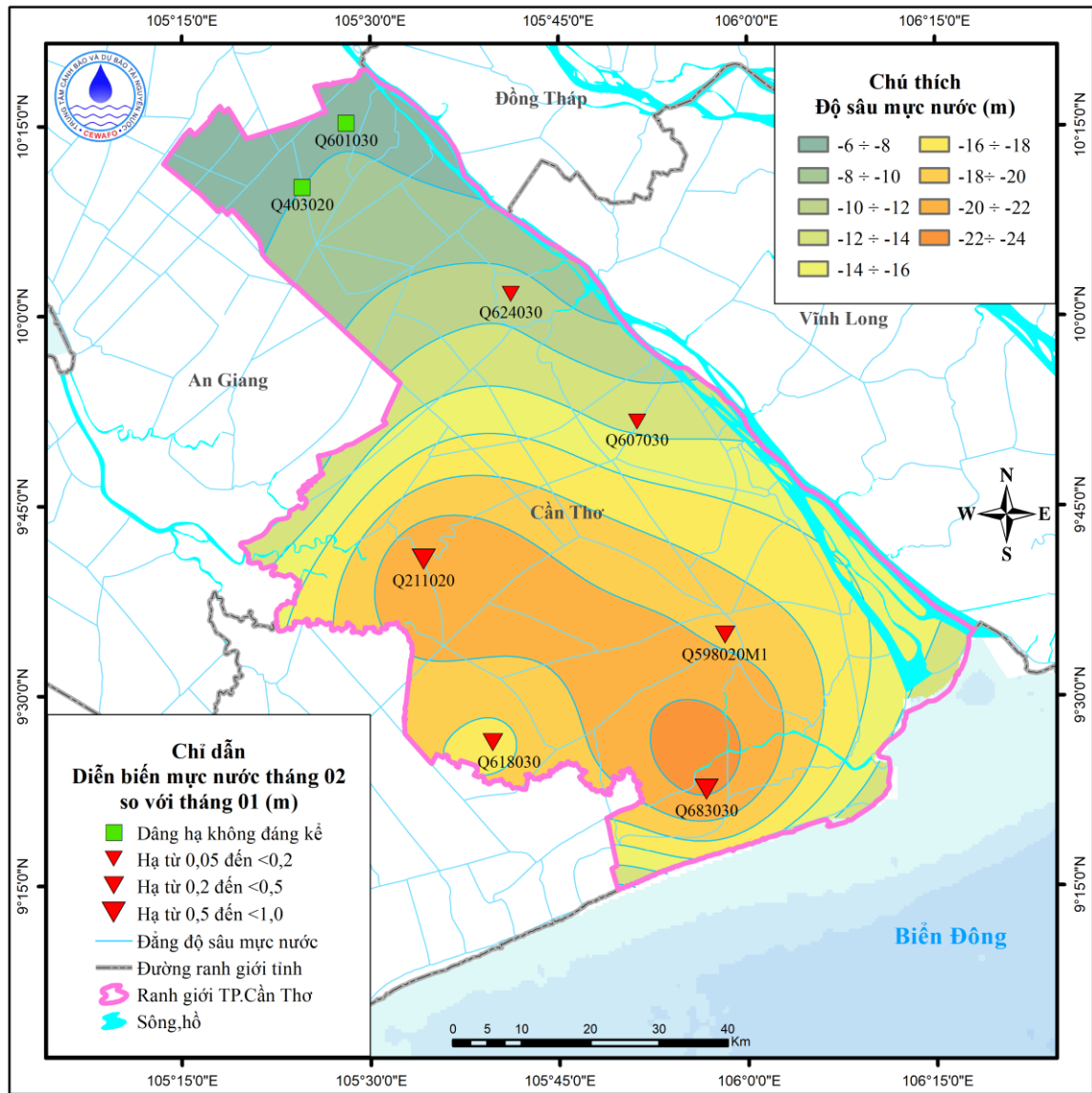
Hình 3. Sơ đồ diễn biến mực nước tháng 02 tầng q_{2-3}
