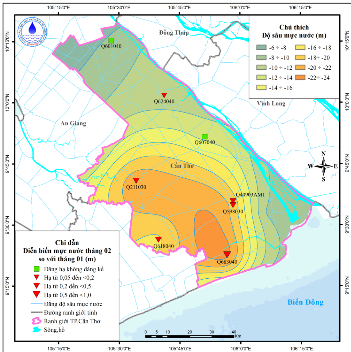
Hình 4. Sơ đồ diễn biến mực nước tháng 02 tầng q_1
