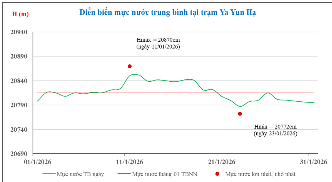
Hình 1. Diễn biến mực nước trung bình ngày tháng 01 năm 2026 tại trạm Ya Yun Hạ
