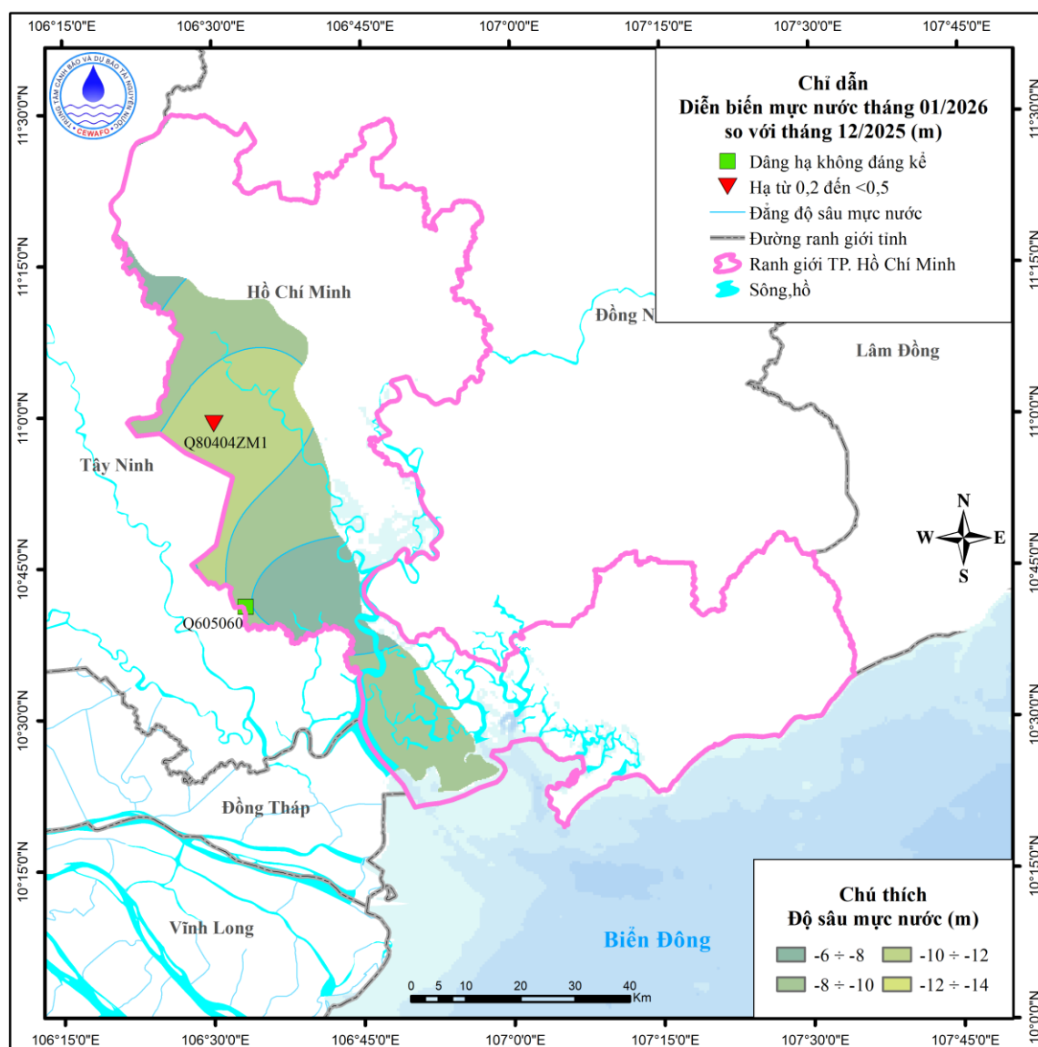
Hình 6. Sơ đồ diễn biến mực nước tháng 01 năm 2026 tầng n_2^1 g) Tầng chứa nước lỗ hổng trong các đá trầm tích Miocene trên ( n_1^3 )
