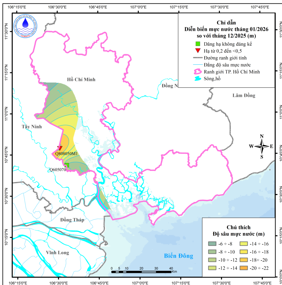
Hình 7. Sơ đồ diễn biến mực nước tháng 01 năm 2026 tầng n_1^3
