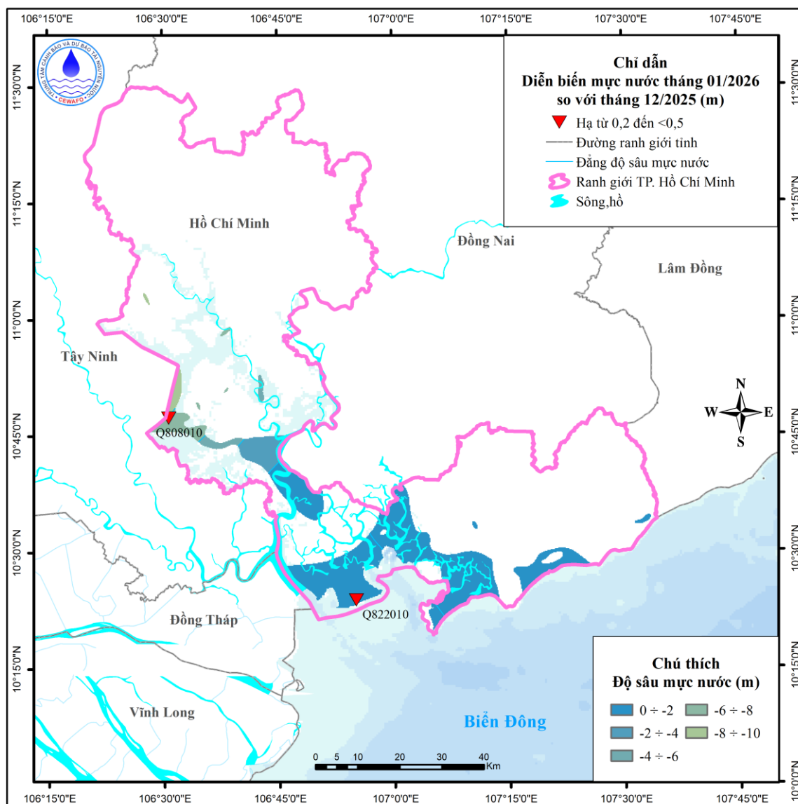
Hình 1. Sơ đồ diễn biến mực nước tháng 01 năm 2026 tầng qh
