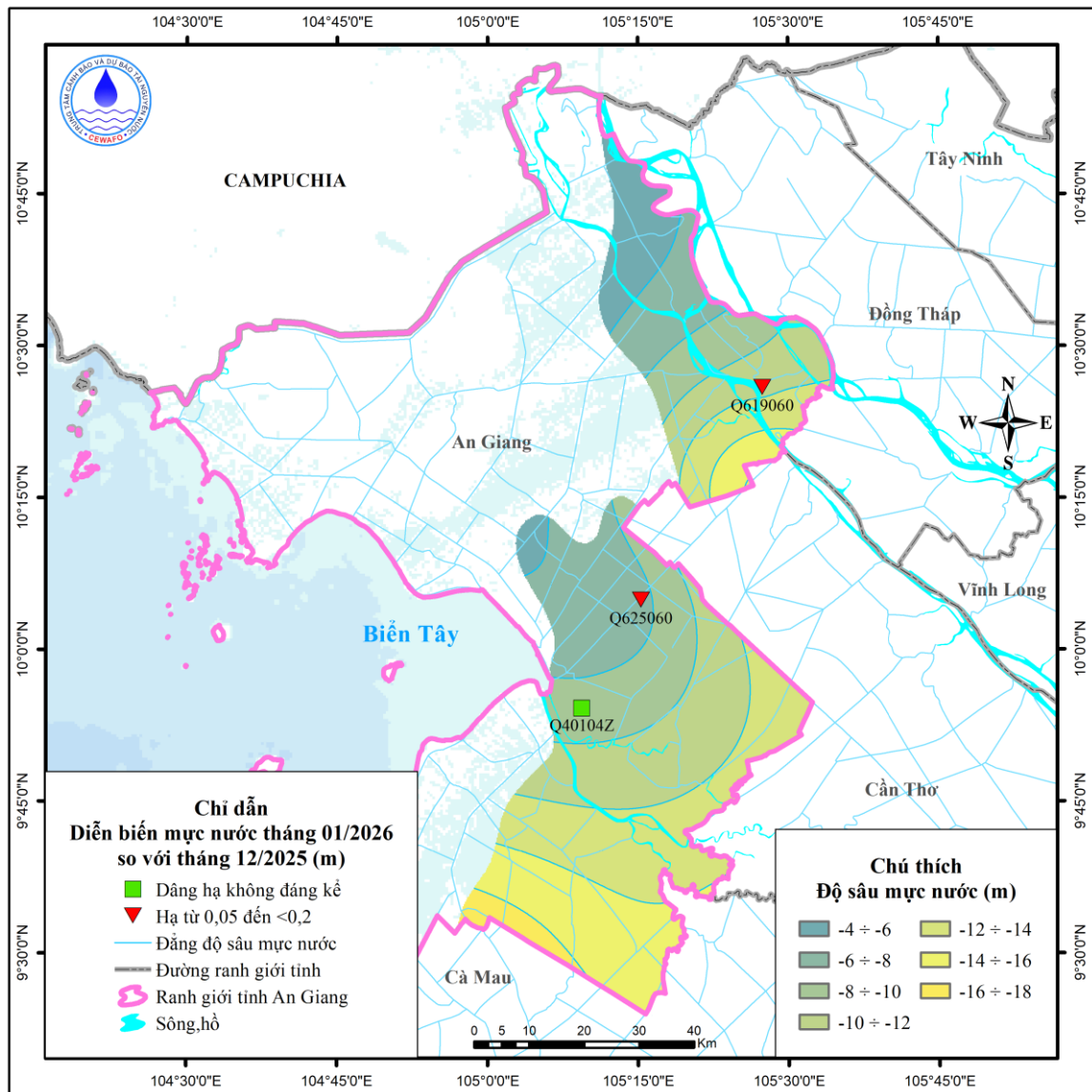
Hình 6. Sơ đồ diễn biến mực nước tháng 01 năm 2026 tầng n_2^I
