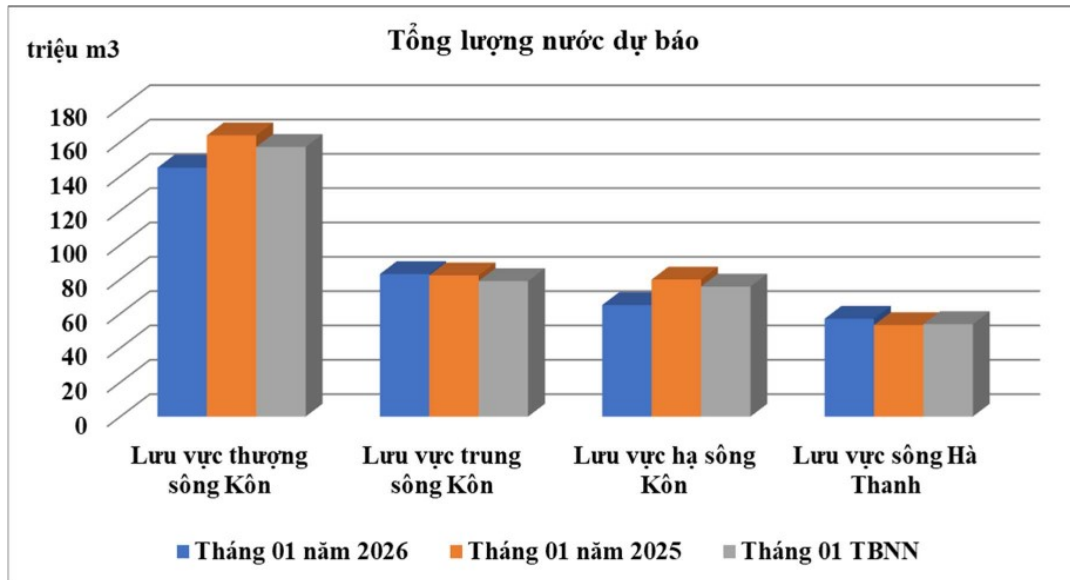
Hình 9. Biểu đồ tổng lượng nước dự báo tháng 01 năm 2026
