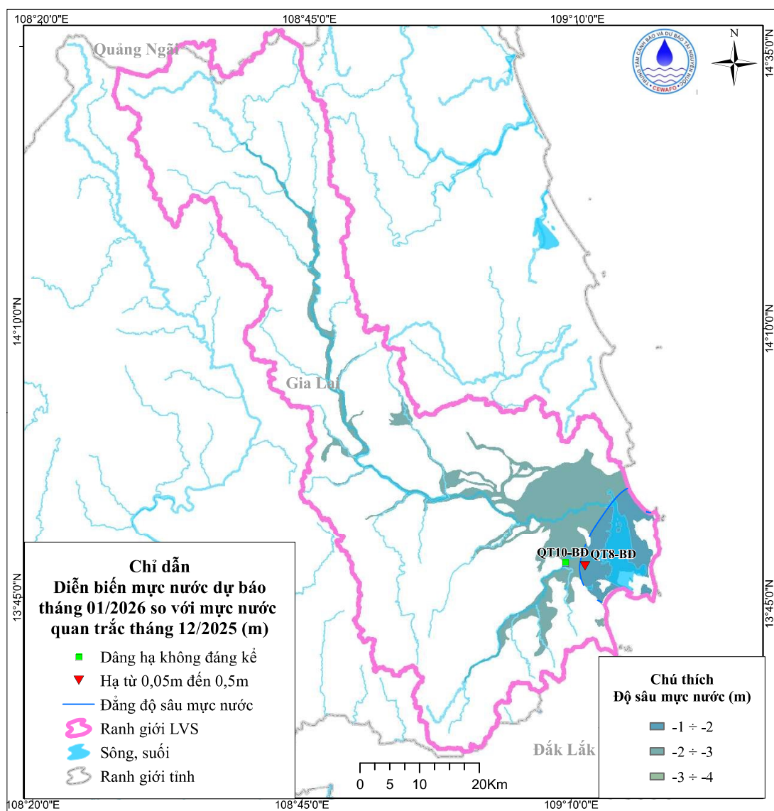
Hình 10. Sơ đồ dự báo diễn biến mực nước tháng 01 năm 2026 tầng qh
