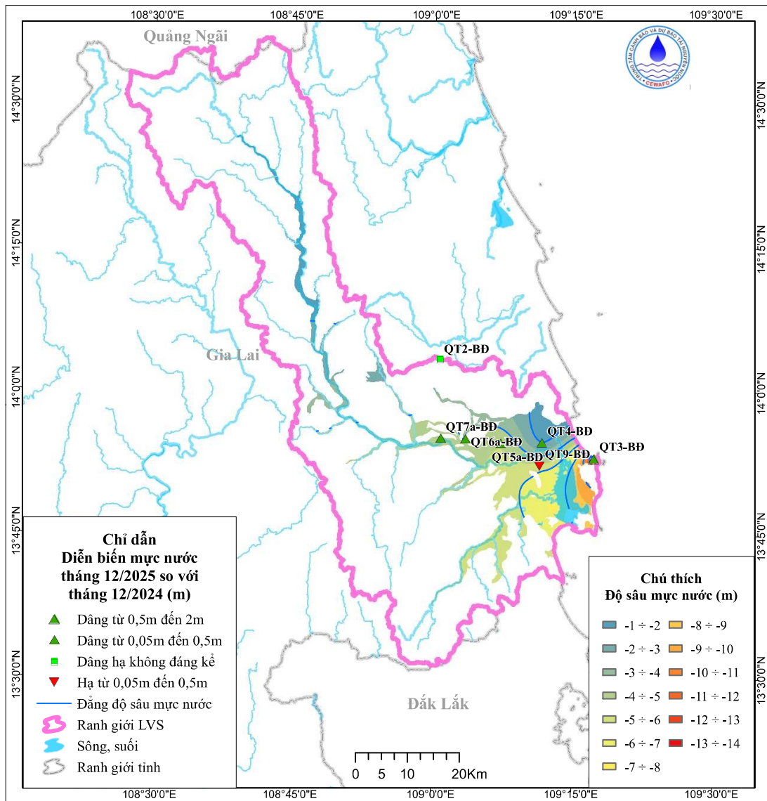
Hình 5. Sơ đồ diễn biến mực nước tháng 12 so với cùng kỳ năm trước
