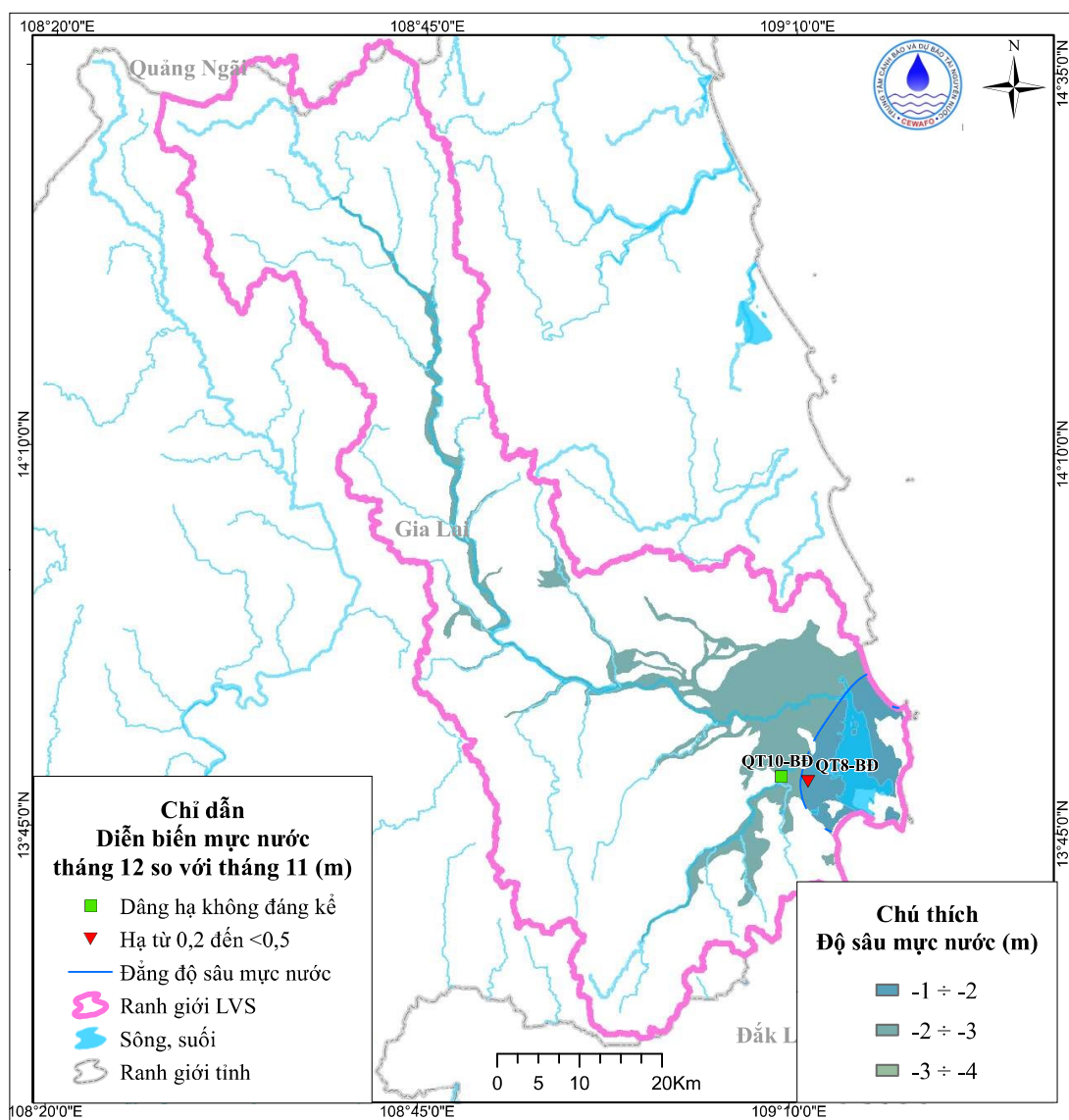
Hình 2. Sơ đồ diễn biến mực nước tháng 12 từng qh
