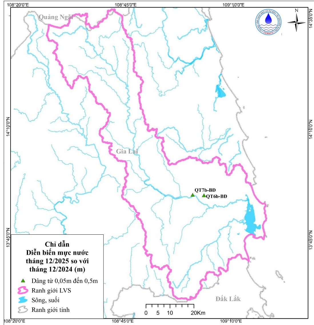
Hình 7. Sơ đồ diễn biến mực nước tháng 12 so với cùng kỳ năm trước
