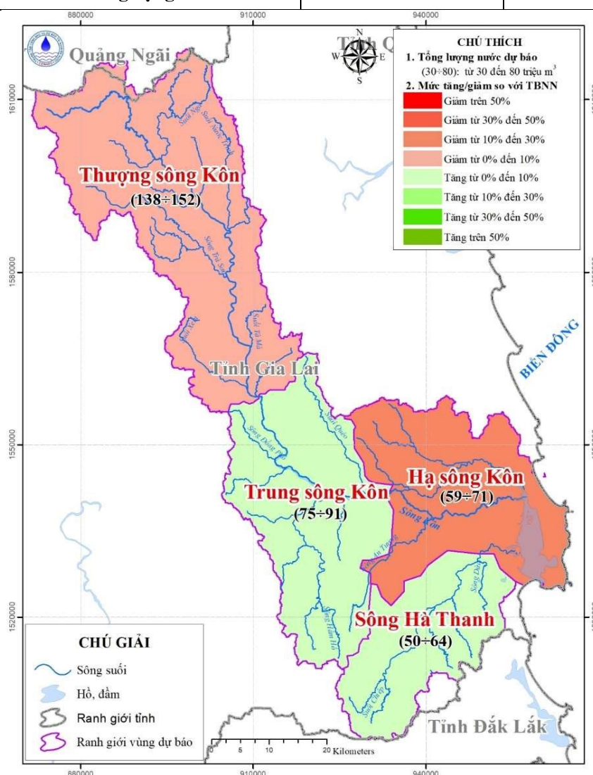
Hình 8. Dự báo tổng lượng nước nội sinh tại các vùng dự báo
