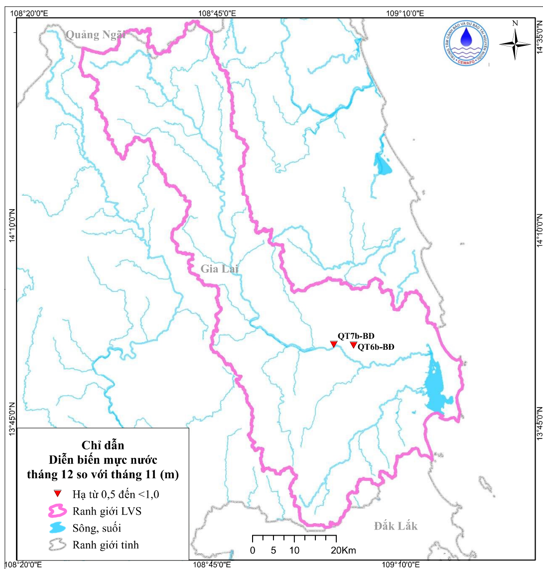
Hình 6. Sơ đồ diễn biến mực nước tháng 12 tăng ar
