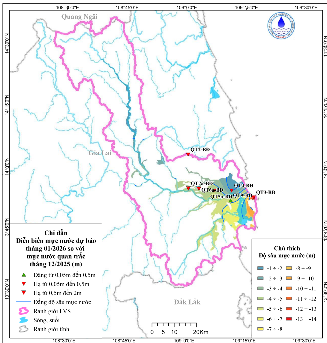
Hình 11. Sơ đồ dự báo diễn biến mực nước tháng 01 năm 2026 tầng qp
