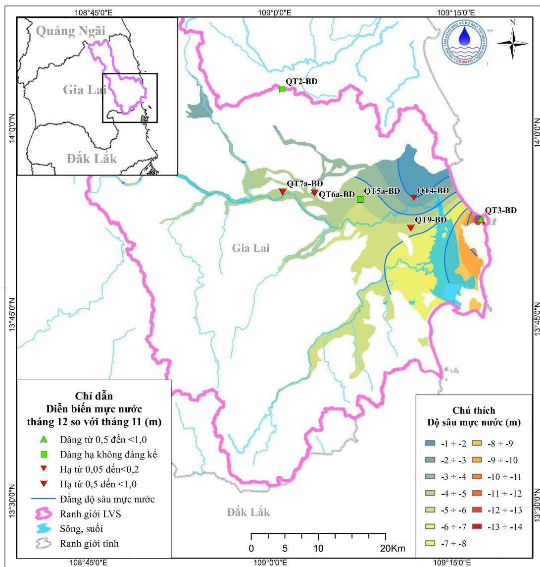
Hình 4. Sơ đồ diễn biến mực nước tháng 12 tầng qp
