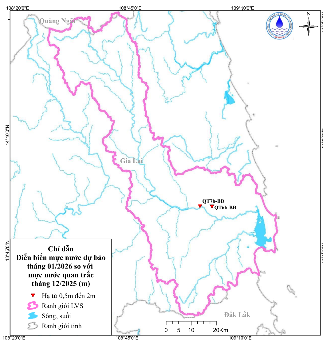
Hình 12. Sơ đồ dự báo diễn biến mực nước tháng 01 năm 2026 tăng ar
