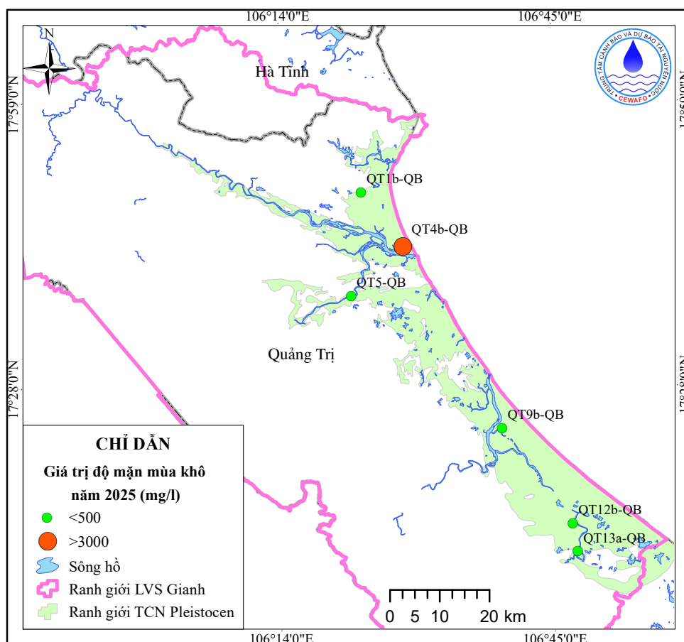
Hình 14. Sơ đồ phân bố giá trị độ mặn mùa khô năm 2025
