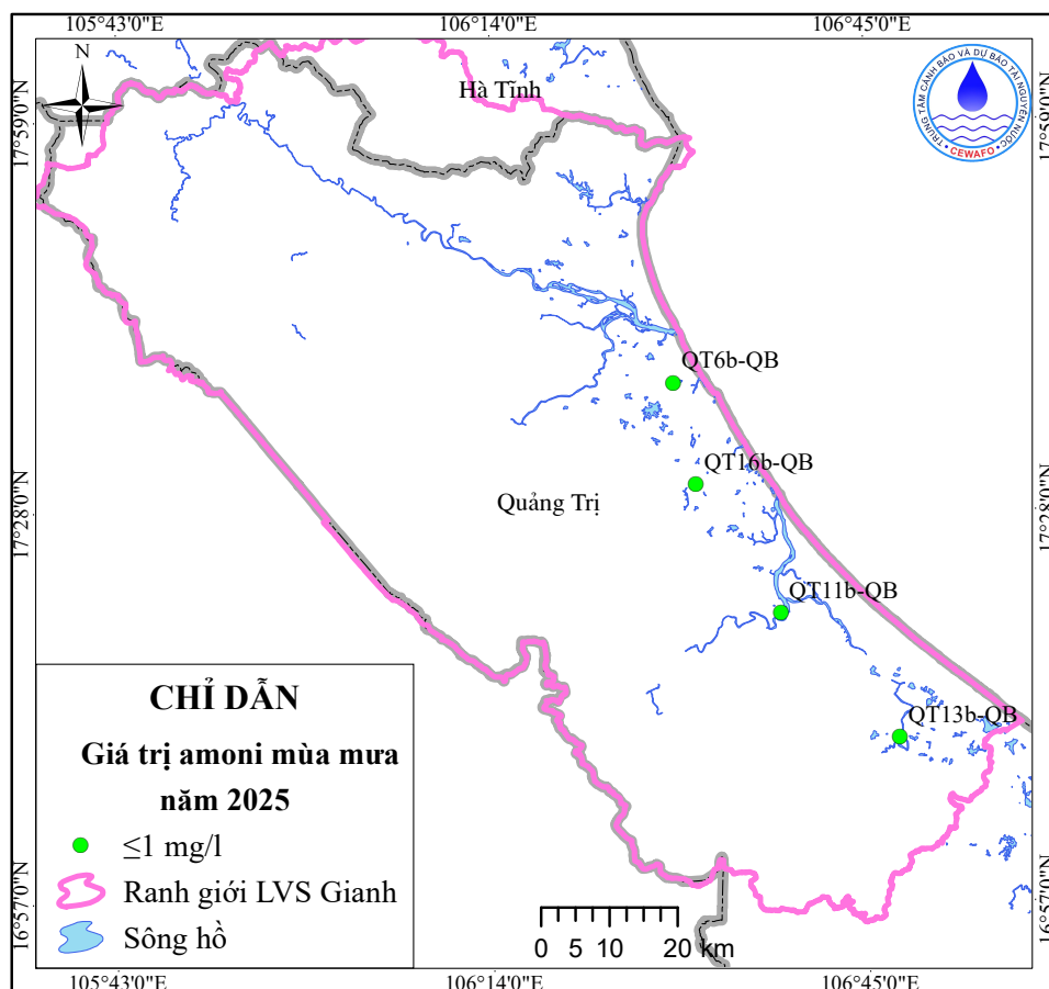
Hình 21. Sơ đồ phân bố giá trị amoni mùa mưa năm 2025
