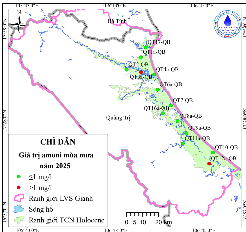
Hình 13. Sơ đồ phân bố giá trị amoni mùa mưa năm 2025
