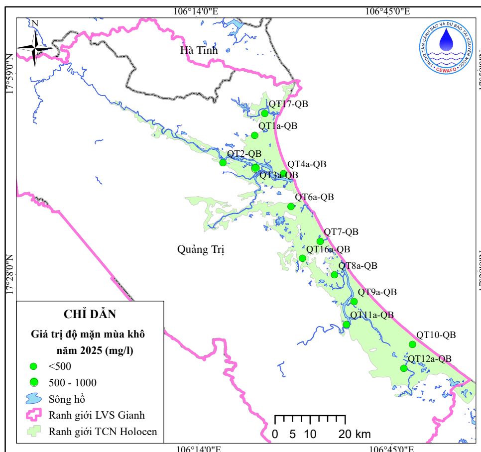
Hình 10. Sơ đồ phân bố giá trị độ mặn mùa khô năm 2025
