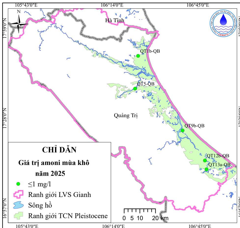
Hình 16. Sơ đồ phân bố giá trị amoni mùa khô năm 2025
