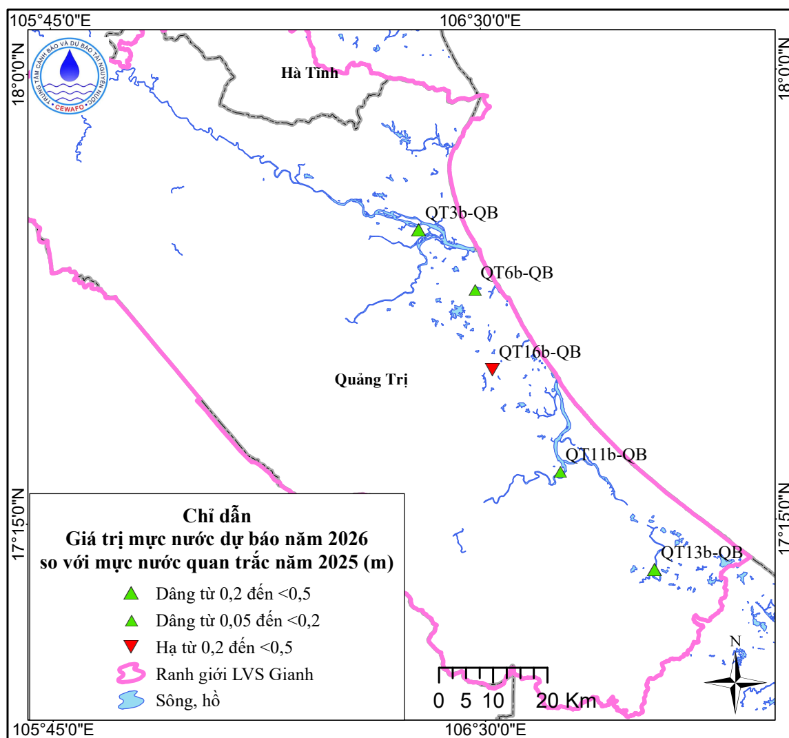
Hình 24. Sơ đồ dự báo diễn biến mực nước tầng d 1
