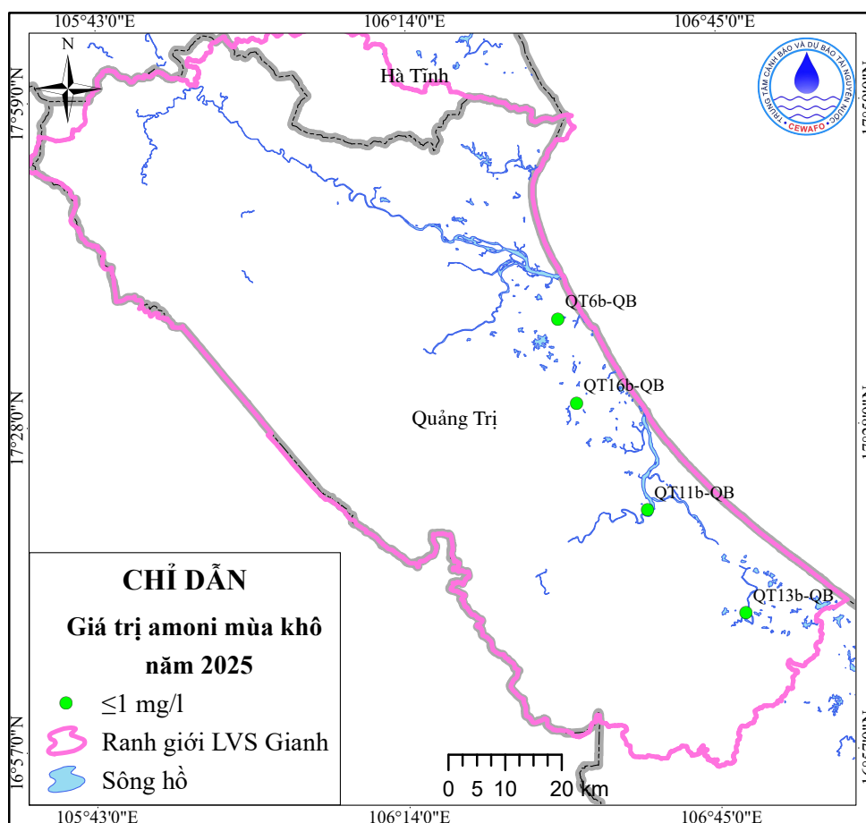
Hình 20. Sơ đồ phân bố giá trị amoni mùa khô năm 2025
