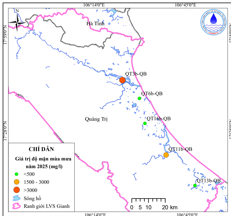
Hình 19. Sơ đồ phân bố giá trị độ mặn mùa mưa năm 2025
