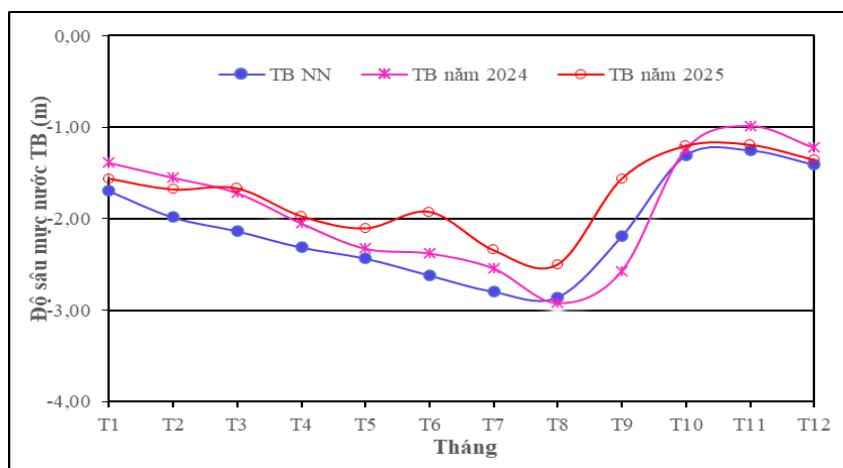
Hình 1. Đồ thị mực nước trung bình tháng năm 2024, 2025 và trung bình nhiều năm
