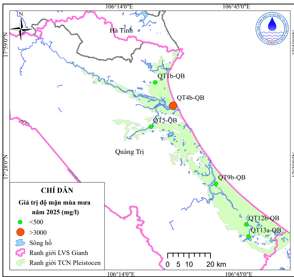
Hình 15. Sơ đồ phân bố giá trị độ mặn mùa mưa năm 2025
