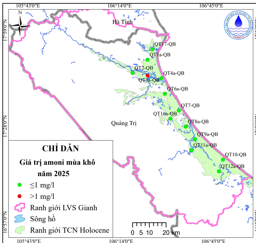
Hình 12. Sơ đồ phân bố giá trị amoni mùa khô năm 2025
