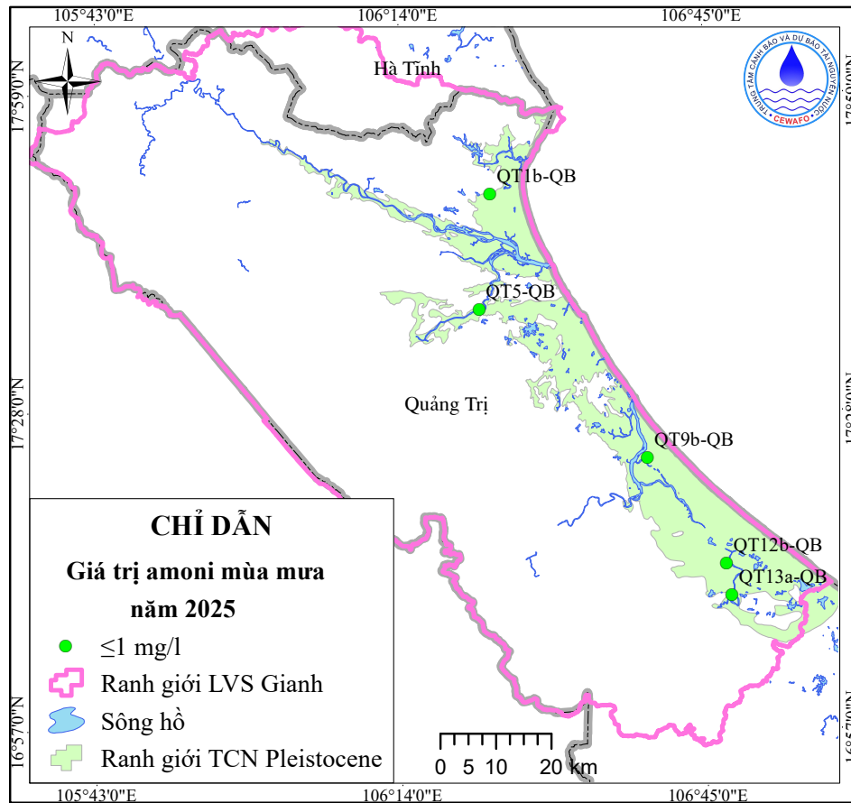
Hình 17. Sơ đồ phân bố giá trị amoni mùa mưa năm 2025
