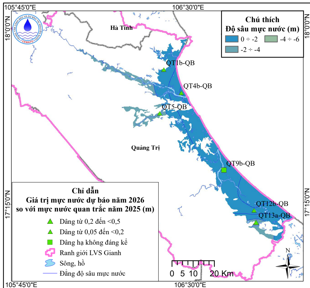
Hình 23. Sơ đồ dự báo diễn biến mực nước tầng q p
