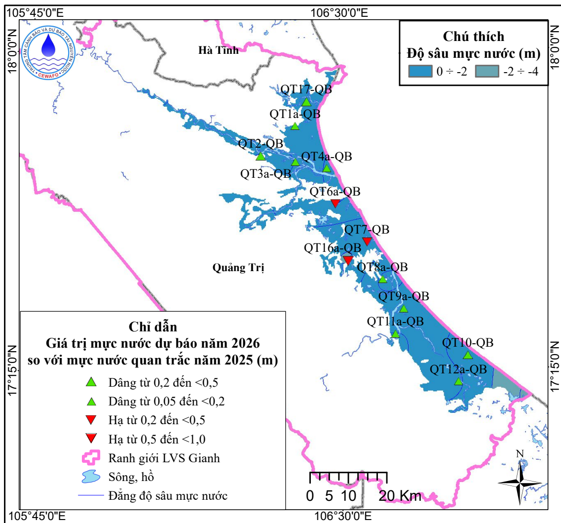
Hình 22. Sơ đồ dự báo diễn biến mực nước tầng qh
