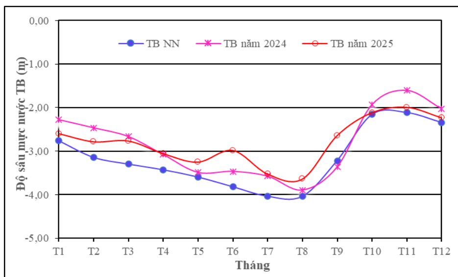
Hình 7. Đồ thị mực nước trung bình tháng năm 2024, 2025 và trung bình nhiều năm
