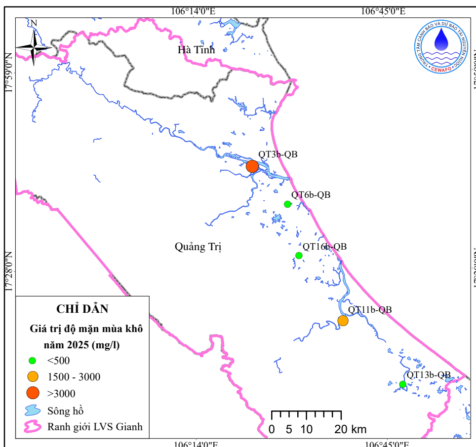
Hình 18. Sơ đồ phân bố giá trị độ mặn mùa khô năm 2025
